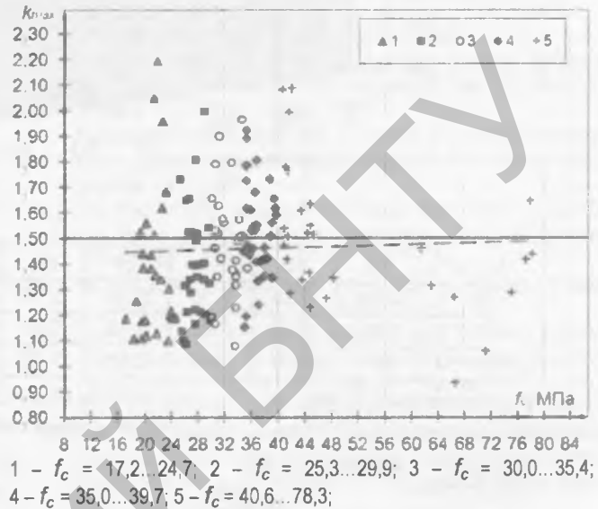
Рис. 3. Зависимость k_{max} от прочности бетона f_c
