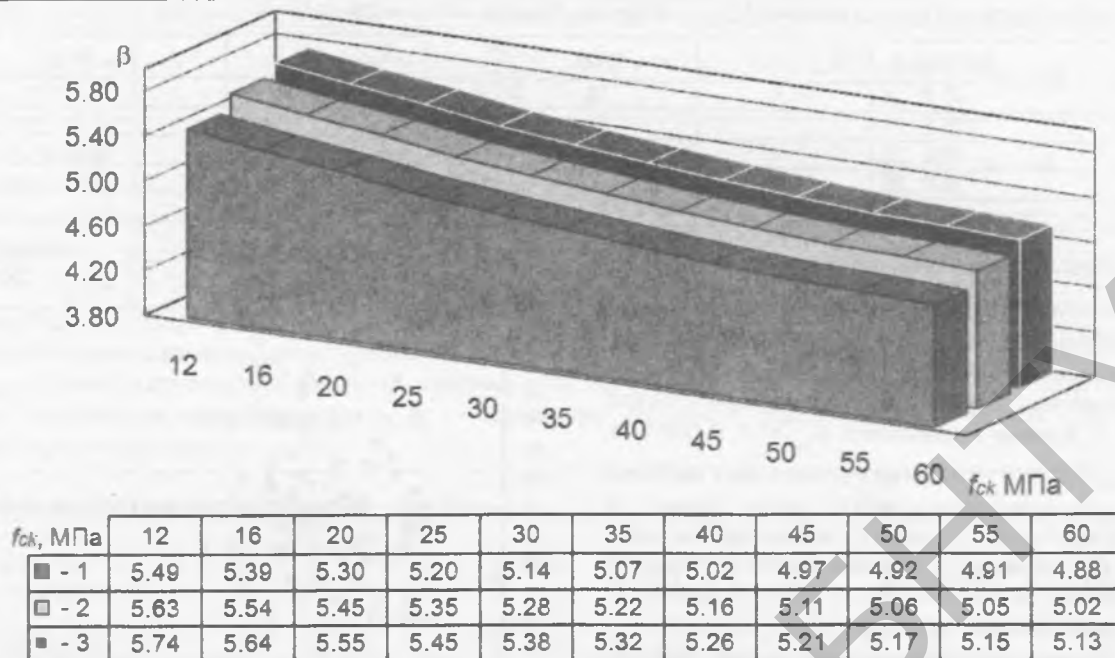
Рис. 4. Зависимость значений индекса надежности \beta от значений прочности бетона f_{ck} при \rho_{sw,min} (при d = 250 мм ( h=300 мм) и проценте продольного армирования \rho = 2\% )
