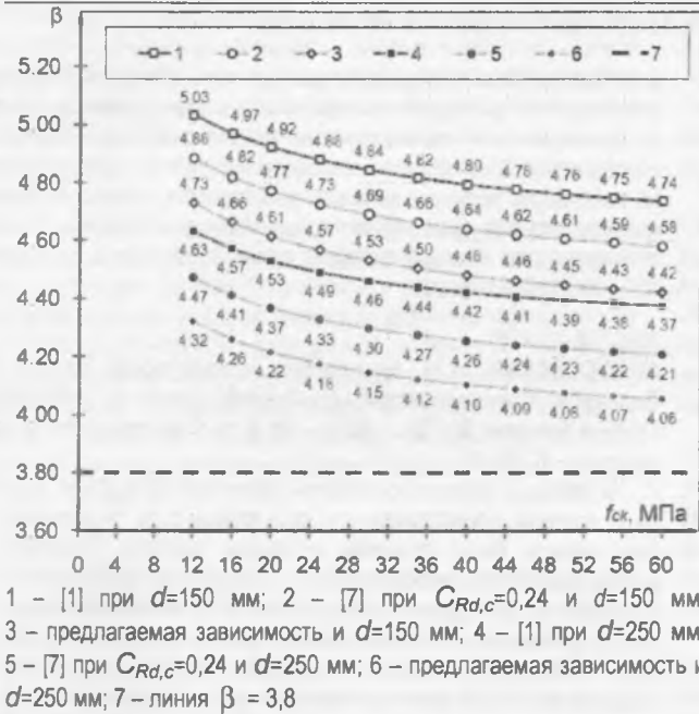
Рис. 6. Зависимость значений индекса надежности \beta от значений прочности бетона f_{ck} при различных значениях рабочей высоты
