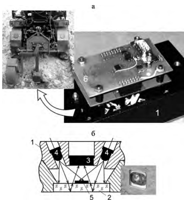
Рис. 1. Конструктивная часть (а) и оптическая схема (б) электронно-оптического модуля интеллектуальной светодетекторной системы: 1 – корпус; 2 – прозрачное окно; 3 – рабочий фотодиод; 4 – светодиоды; 5 – контрольный фотодиод; 6 – электронная схема
