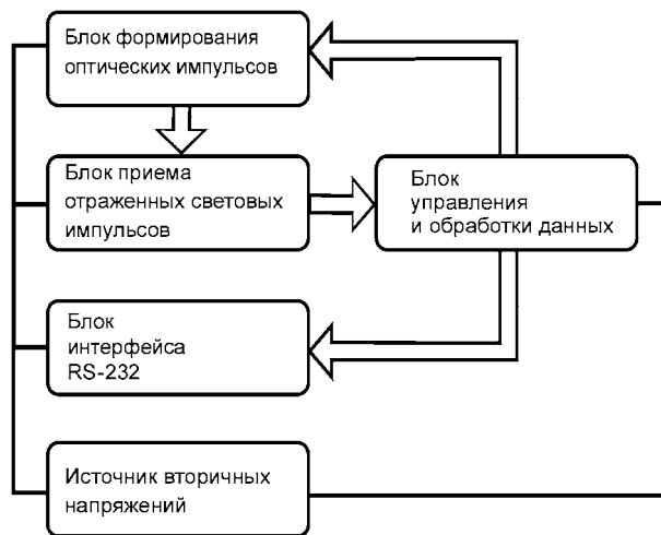
Рис. 2. Структурная схема интеллектуального сенсорного модуля для светоцветового контроля почвы
