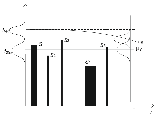
Рис. 2. Схема процесса нагружения конструкции реальной нагрузкой и ее деградации во времени
