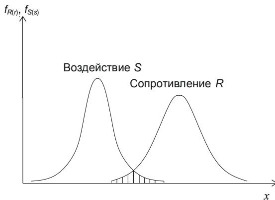
Рис. 1. Схема взаимодействия распределений вероятностей обобщенного сопротивления и обобщенного воздействия
