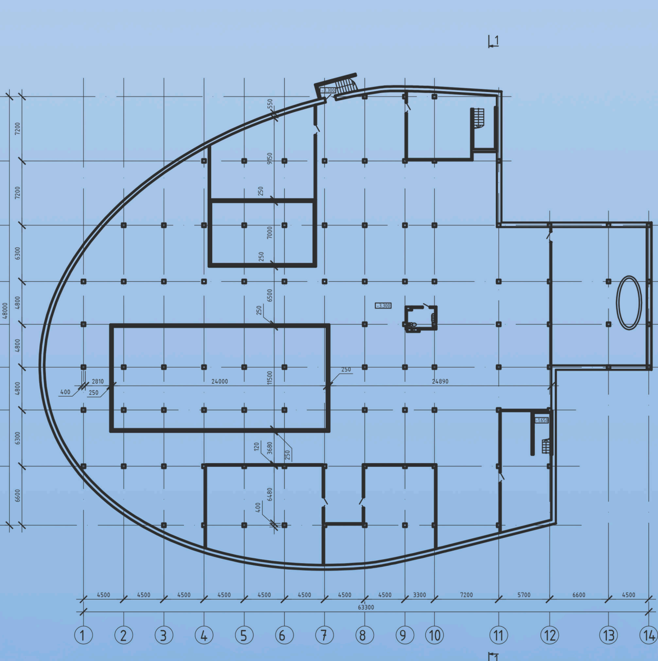
План на отметке -3.300
