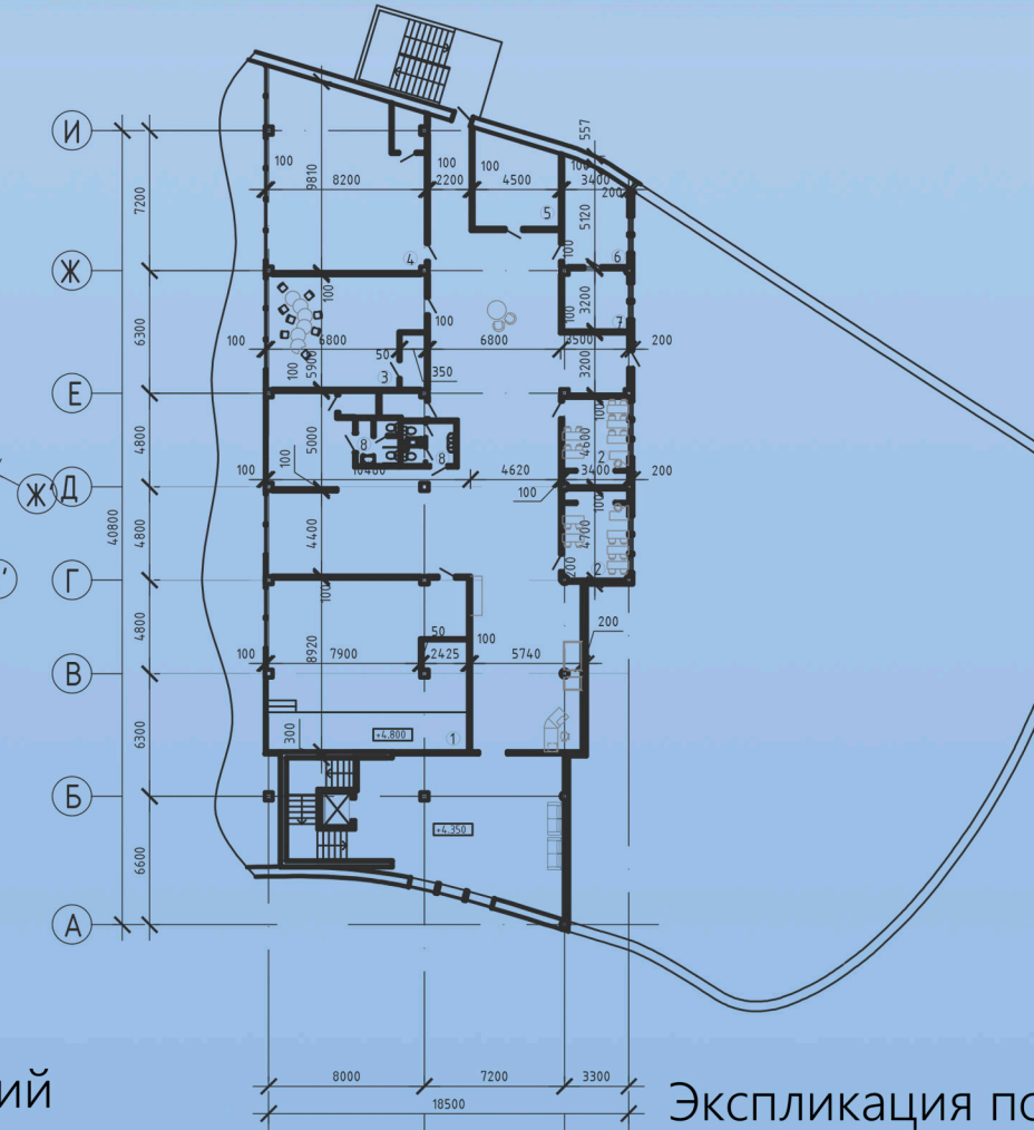
План на отметке +4.350
