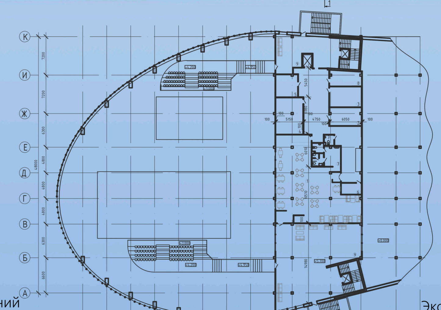
План на отметке +5.700
