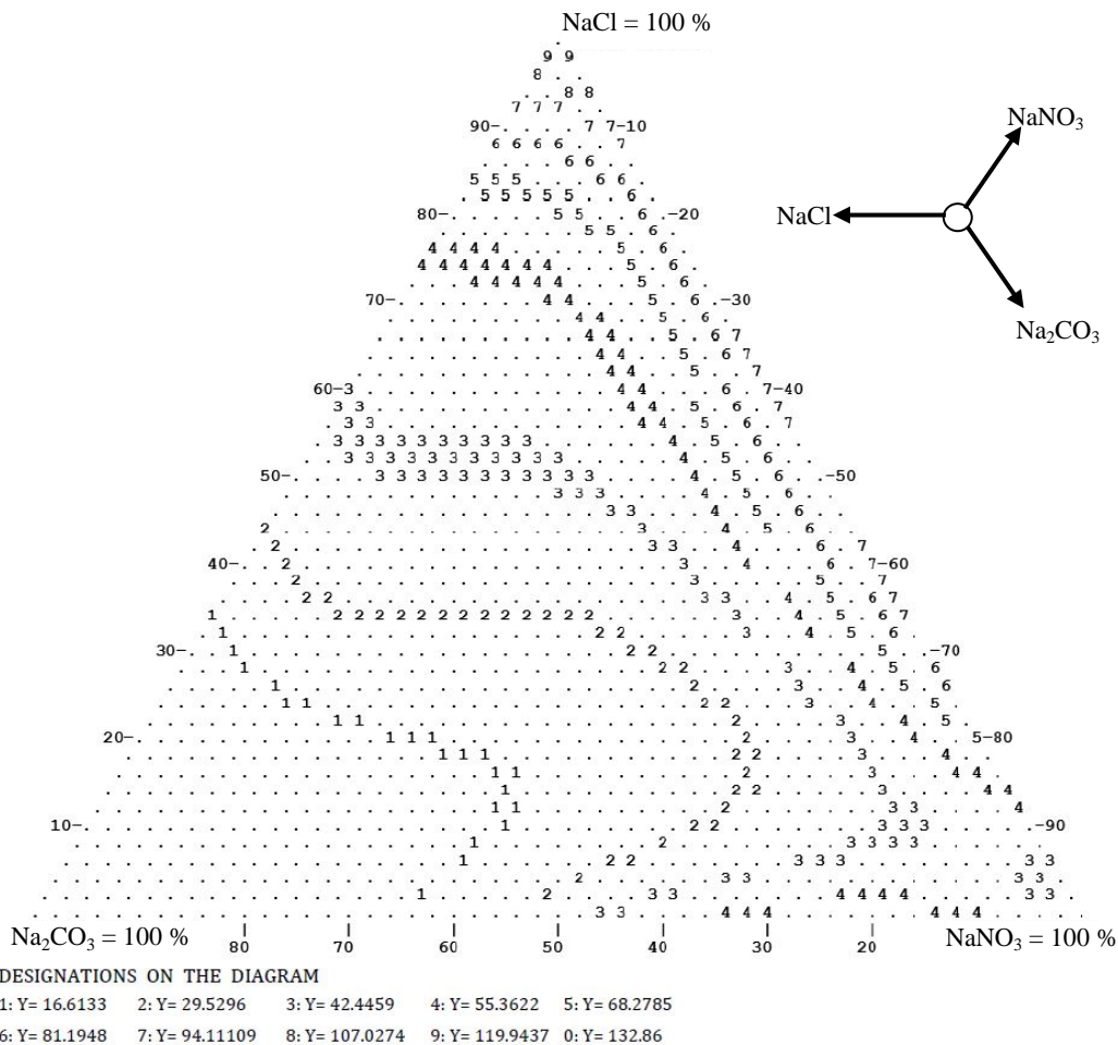
Рис. 3. Показатель коррозии (µм/год) в растворе солей \text{NaNO}_3 , \text{NaCl} и \text{Na}_2\text{CO}_3 в зависимости от состава раствора Fig. 3. Corrosion index ( \mu\text{m}/\text{year} ) in solution of \text{NaNO}_3 , \text{NaCl} and \text{Na}_2\text{CO}_3 salts, depending on composition of solution
