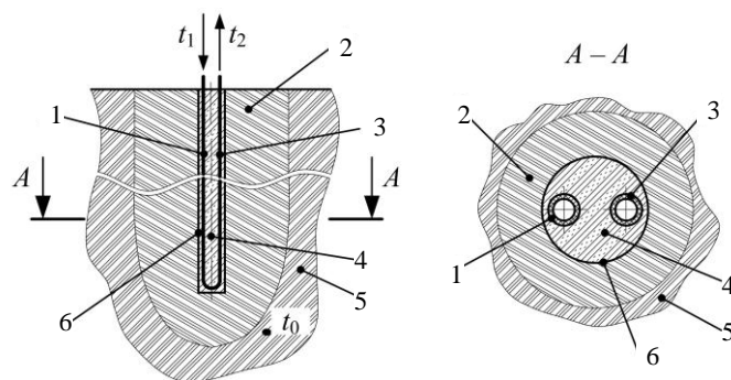
Рис. 1. Вертикальный грунтовый теплообменник: 1 – нисходящая ветвь U-образной трубы; 2 – область грунта, вступающего в тепловое взаимодействие с ВГТО; 3 – восходящая ветвь U-образной трубы; 4 – заполнитель скважины; 5 – область грунта, не вступающего в тепловое взаимодействие с ВГТО; 6 – поверхность скважины
