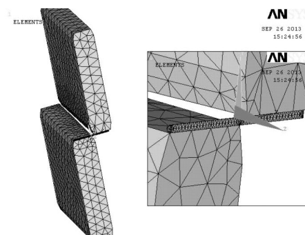
Конечно-элементная модель ножей для рубки фибры
