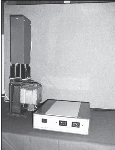
Прибор магнитного неразрушающего контроля структуры чугуновых изделий массового производства «МАКСИ – П (портативный)»
