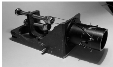
Рисунок 2 – Экспериментальный вариант приспособления для придания проволоки зигзагообразной формы
