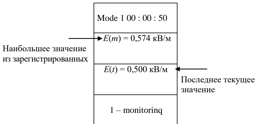
Рис. 7.3. Изображение экрана прибора СТ-01
