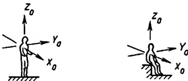
Рис. 6.1. Направление координатных осей при действии вибрации
