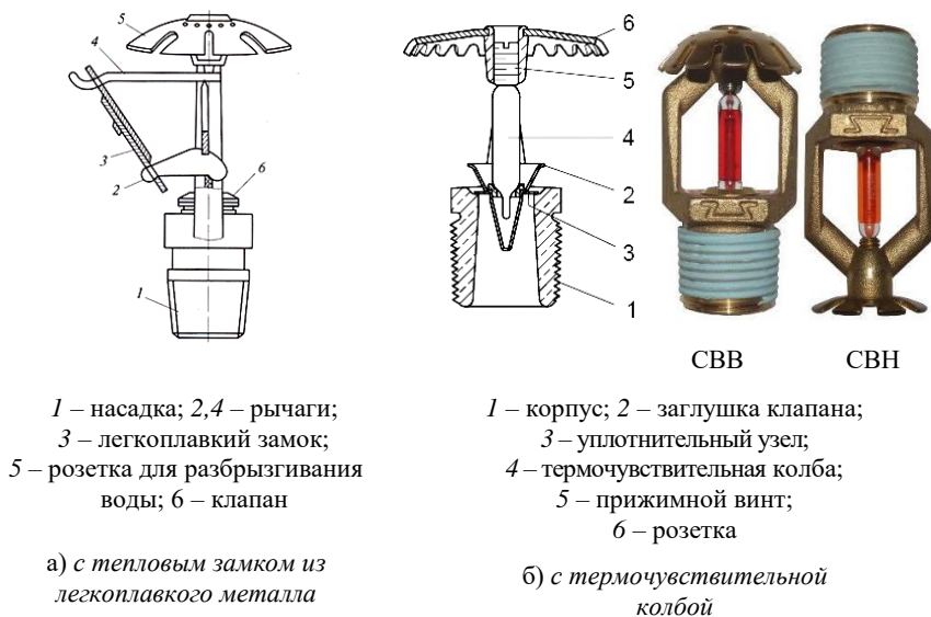
Рис. 8.6. Спринклерные оросители
