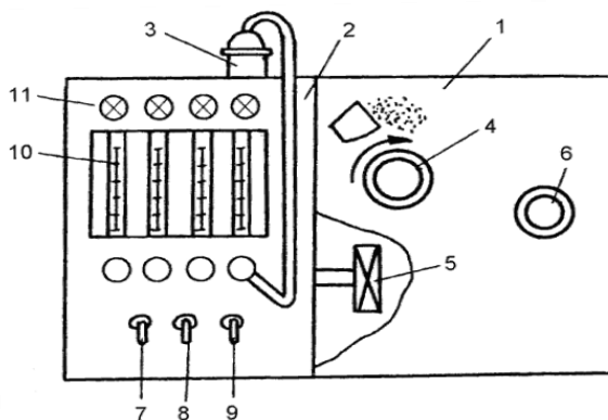
Рис. 4.2. Экспериментальная установка:
