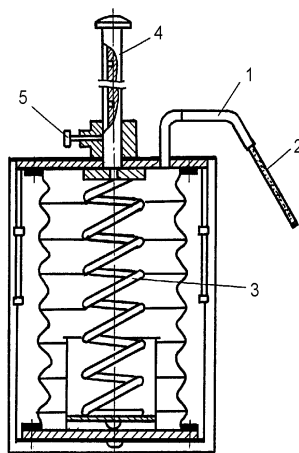
Рис. 4.1. Газоанализатор УГ-2:
