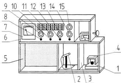
Рис. 5.2. Схема экспериментальной установки:
