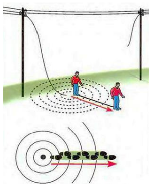
Рис. 9.7. Перемещение в зоне шагового напряжения
