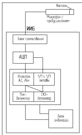
Рис. 5.3. Схема шумомера «Октава-101А»
