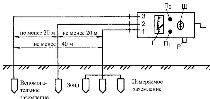
Рис. 1.3. Схема измерения сопротивления заземляющих устройств
