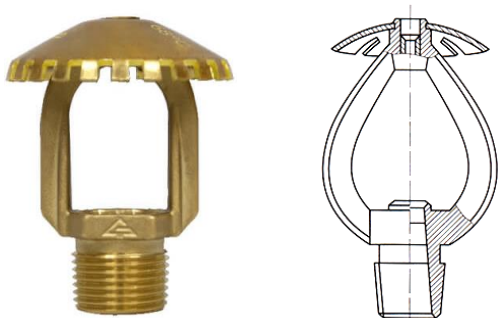
Рис. 8.7. Дренчерный ороситель
