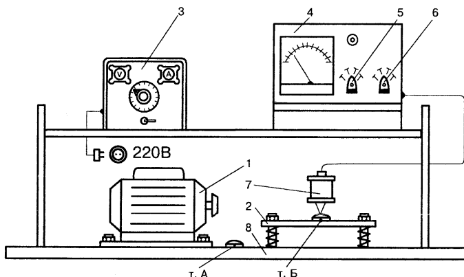
Рис. 6.2. Экспериментальная установка:
