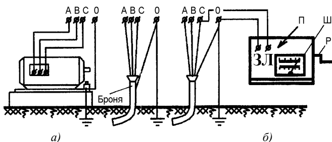
Рис. 1.4. Схема измерения сопротивления изоляции электроустановок
