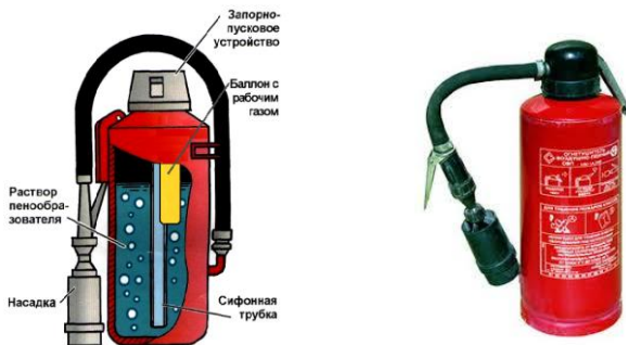
Рис. 8.4 Огнетушитель воздушно-пенный
