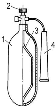
1 – стальной баллон; 2 – вентиль; 3 – сифонная трубка; 4 – раструб
