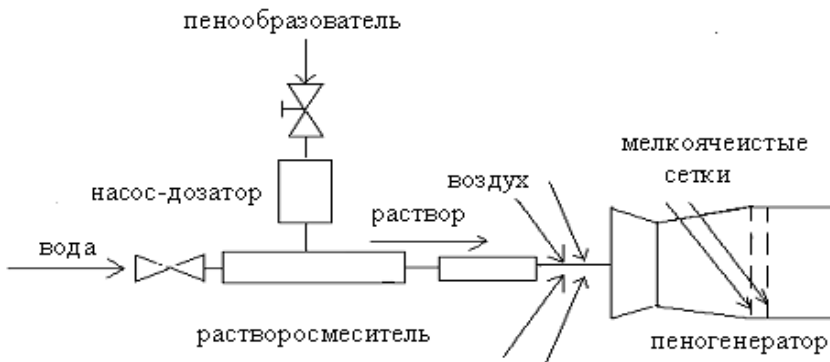
Рис. 8.1. Схема получения воздушно-механической пены
