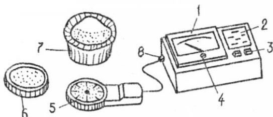
Рис. 2.1. Люксметр Ю-116:
