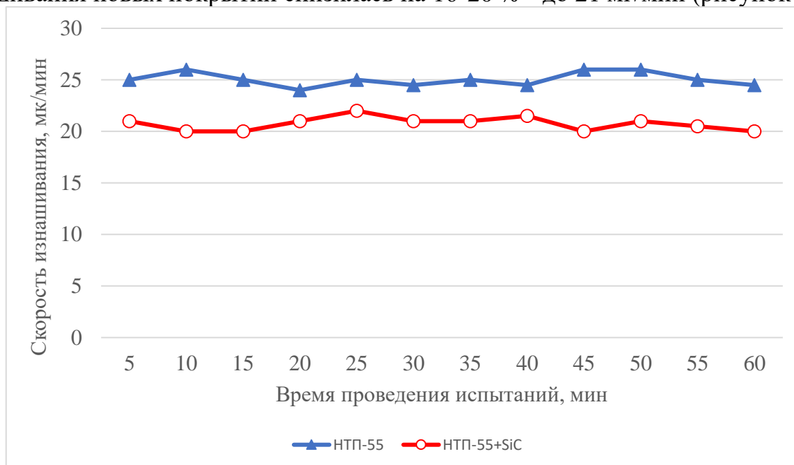
Рисунок 3 – Скорость изнашивания образцов с покрытиями, мг/мин
