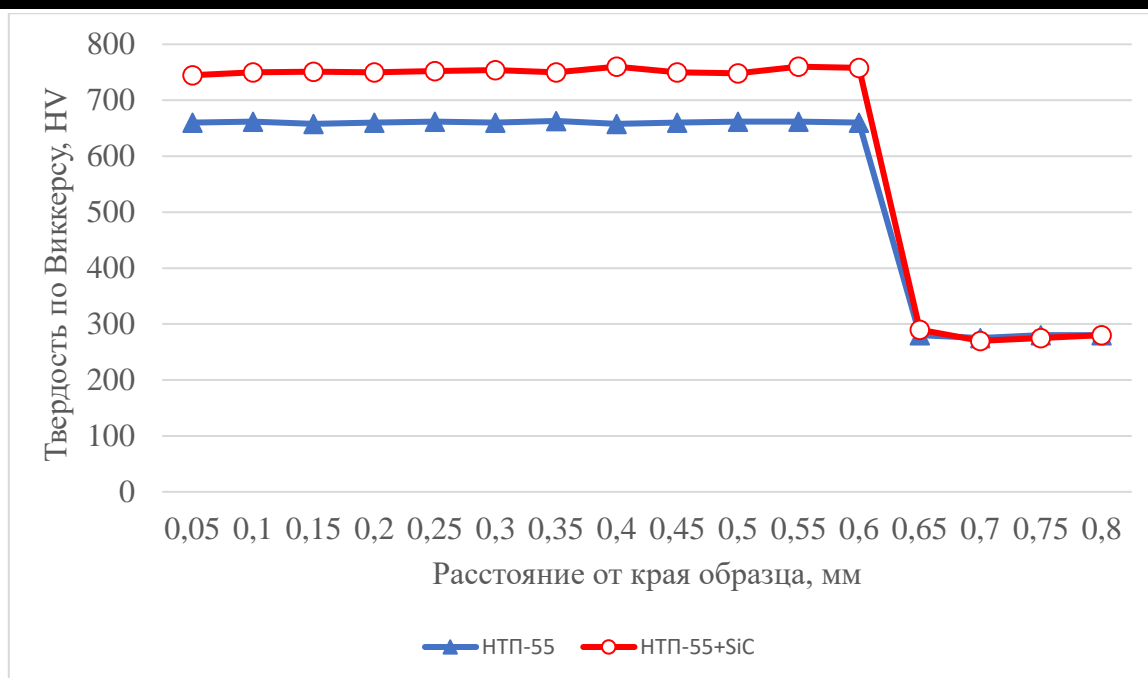
Рисунок 2 – Изменение микротвердости покрытия, HV, по глубине образца
