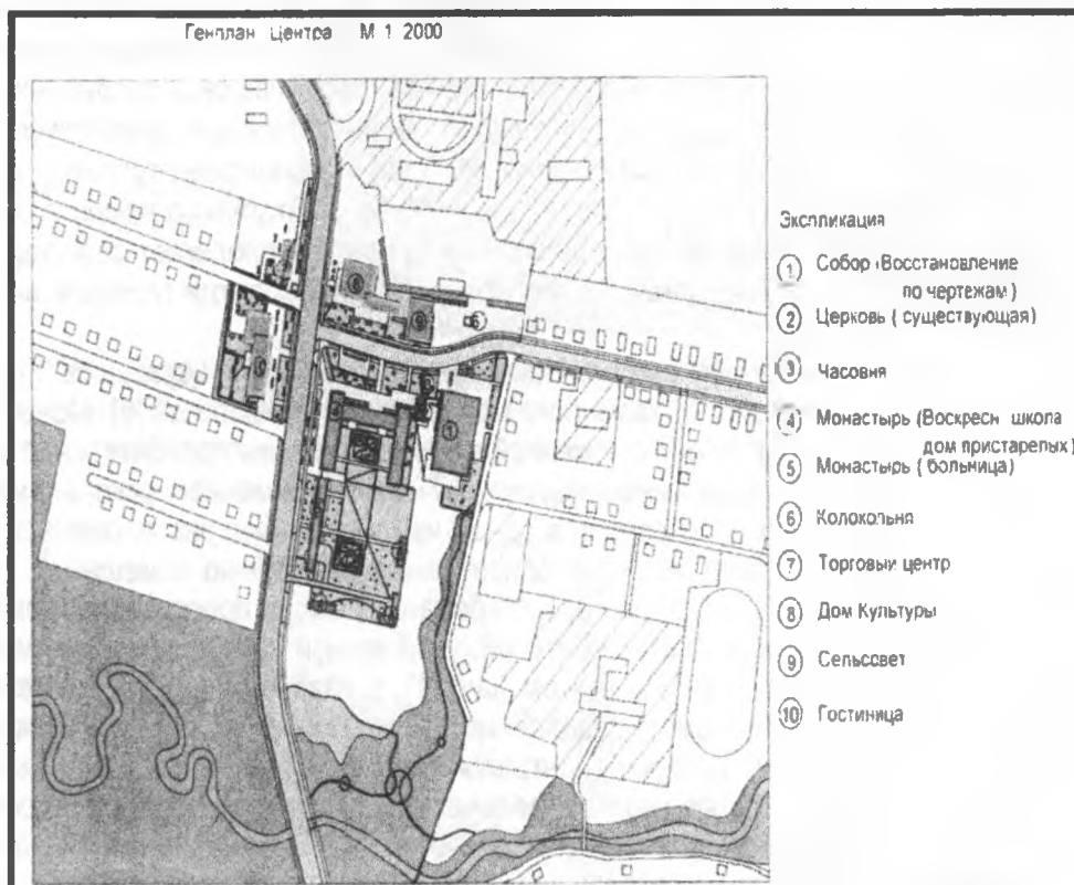
Рисунок 4 – Генплан центра
