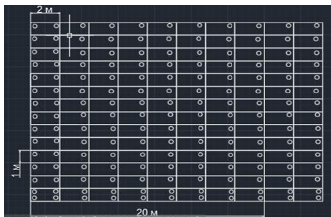
Рис. 1. Принцип расположения опорных ног подиума
