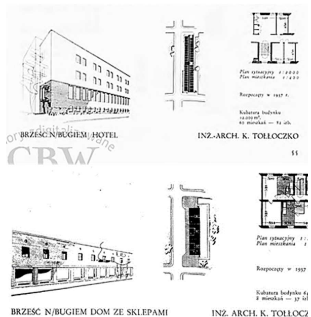
Рис. 4. Застройка поселка Траугуттово (общественные здания): гостиница со столовой и встроенным детским садом и магазин с квартирами для работников [7, с. 55]
