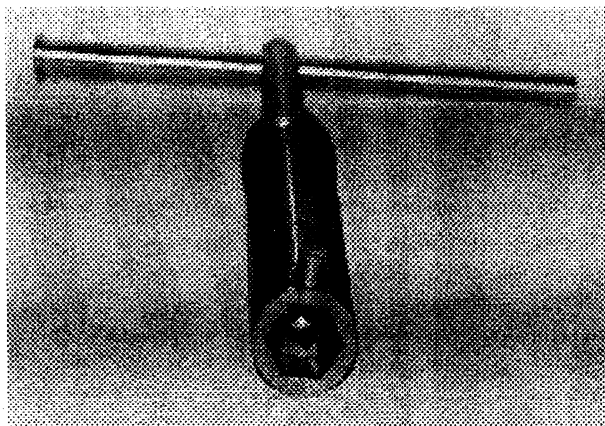
Рис.2. Ключ для демонтажа ведущих колес грузовых автомобилей ЗИЛ и ГАЗ
