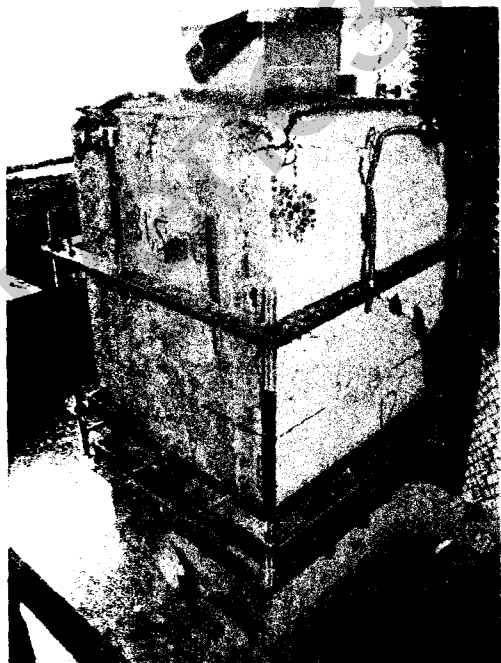
Рис. 1. Общий вид испытаний и характер разрушения образца при передаче нагрузки через штампы сечением 120x120 мм
