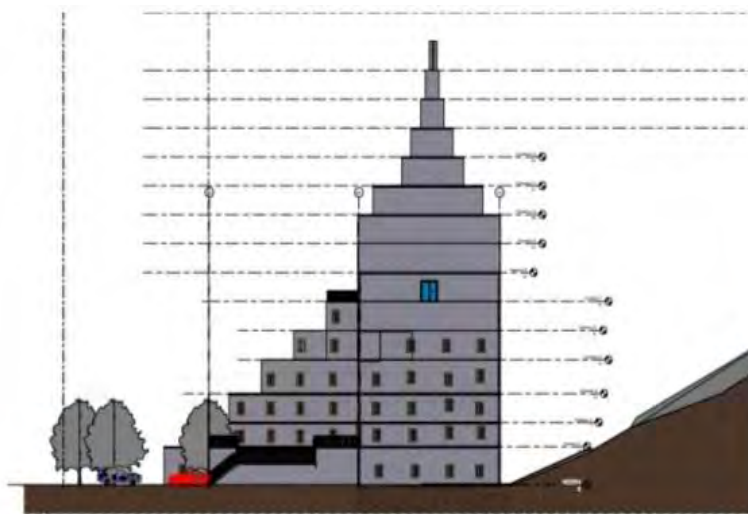
Рисунок 7 – Восточный фасад
