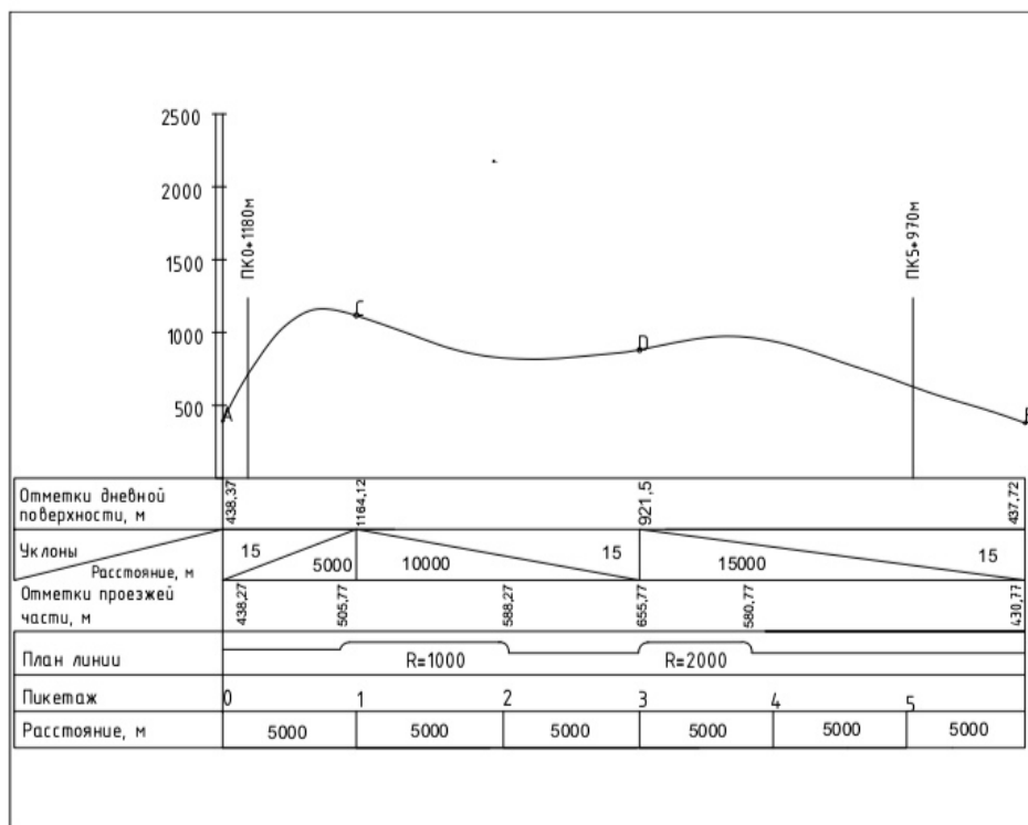
Рисунок 2 – Продольный профиль трассы
