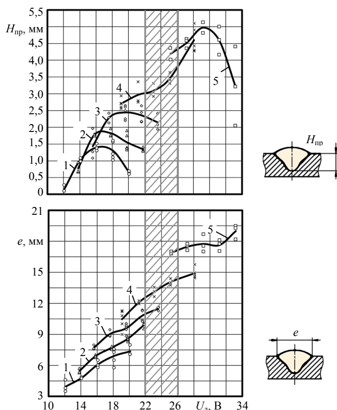
Рис. 3. Графические зависимости глубины проплавления основного металла ( H_{пр} ) и ширины валика наплавленного металла ( e ) от напряжения на дуге ( U_d ) при различном значении силы тока ( I_{св} ): 1 – I_{св} = 100 А; 2 – 150; 3 – 200; 4 – 250; 5 – 300 А
