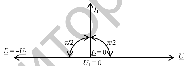
Рис. 5. Векторная диаграмма холостого хода системы передачи
