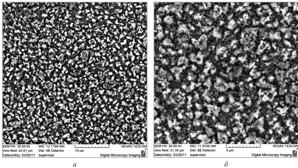
Рис. 2. Структура литой БрХ1, полученной при введении лигатуры в расплав: a – \times 5000 ; б – \times 10000
