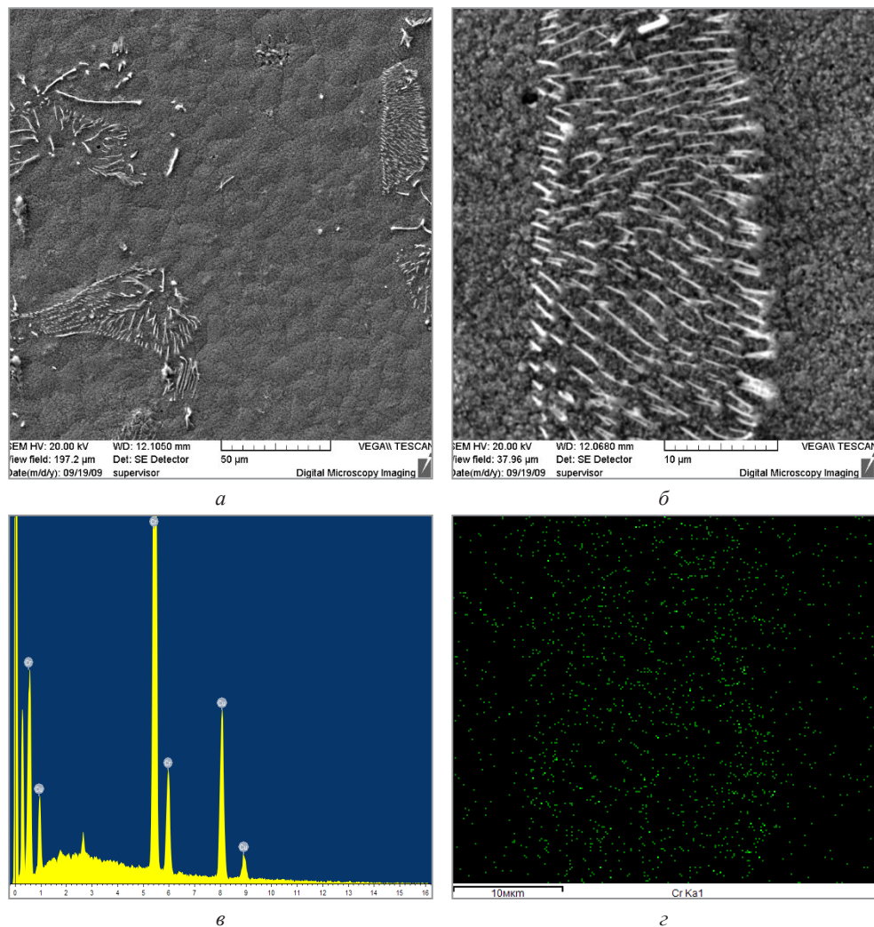
Рис. 3. Структура литой БрХ1 ( a , б ) и распределение Cr при сканировании по площади ( г ): выдержка 2 мин
