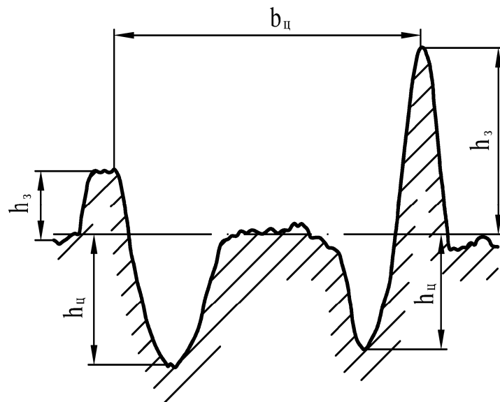
Рис. 12. Формы поперечного сечения микроцарапины, полученной при микроцарапании поверхности образца напльваами металла с различной высотой режущих кромок
