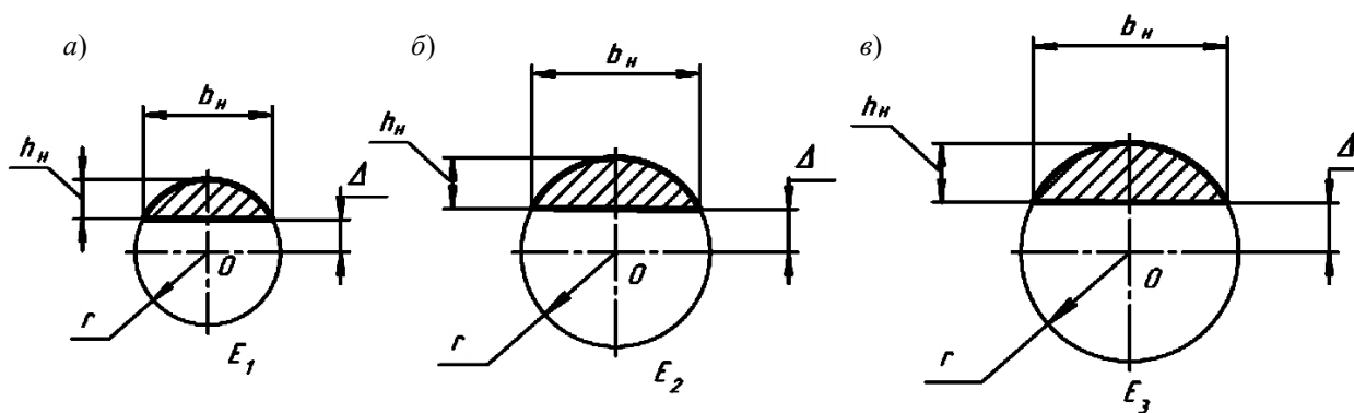
Рис. 4. Схематическое представление изменения формы кругового сегмента в диаметральном сечении напыла металла в зависимости от энергии разряда: а – при E_1 ; б – при E_2 ; в – при E_3 ( E_1 < E_2 < E_3 )
