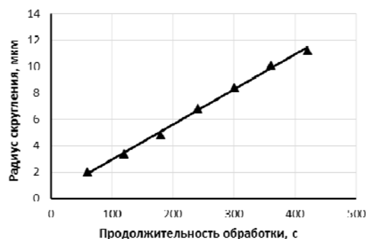
Рисунок 1 – Влияние продолжительности обработки на изменение шероховатости поверхности образцов (а) и на изменение радиуса скругления (б)
