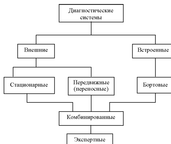
Рис. 1. Классификация диагностических систем автомобилей по расположению технических средств диагностирования
