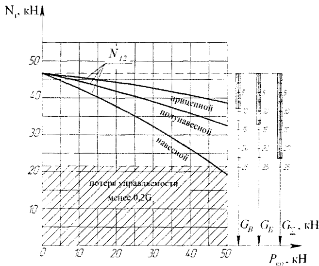
Рис. 1. Номограмма для определения веса балластных грузов при различных способах агрегирования трактора «БЕЛАРУС 3022»
