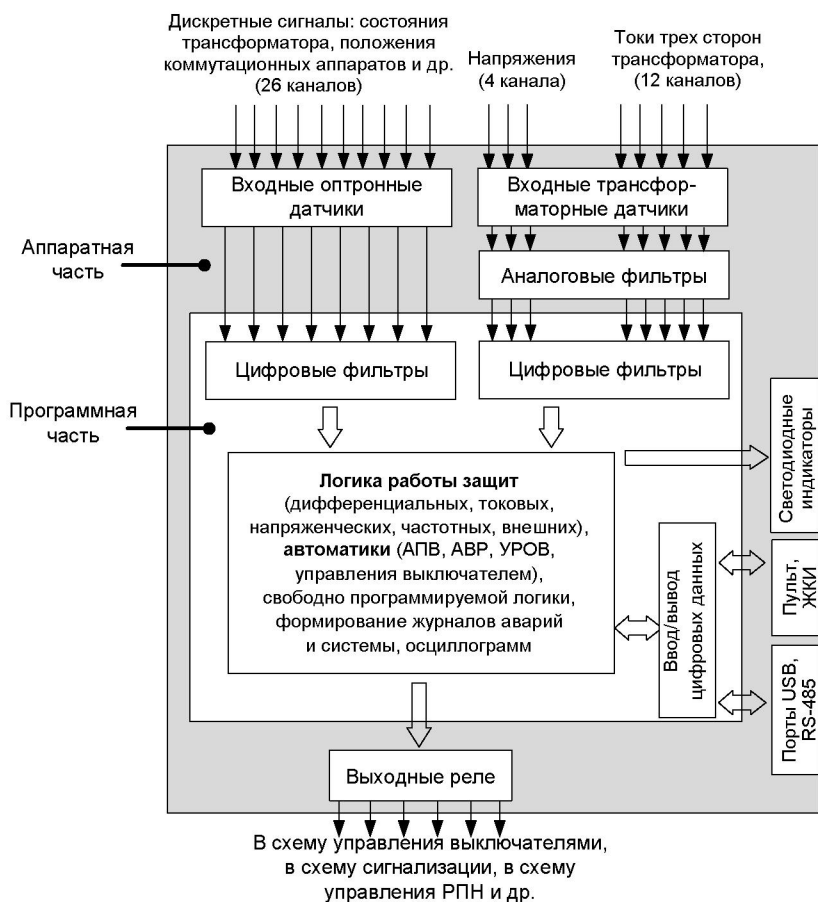
Рис. 1. Структура терминала MP801
