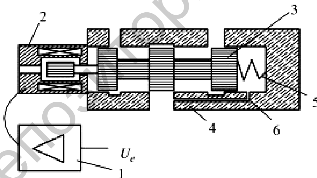
Рис. 2. Устройство ПЭМК давления SMC VER3121: 1 – управляющая цепь; 2 – пропорциональный электромагнит; 3 – золотник; 4 – корпус клапана; 5 – пружина; 6 – пневматическая цепь обратной связи
