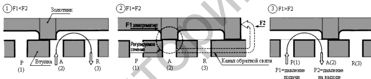
Рис. 3. Упрощенная схема работы пропорционального ЭМК VER3121: P – питающая магистраль (вход клапана); A – выход клапана (к силовому цилиндру); R – выход в атмосферу
