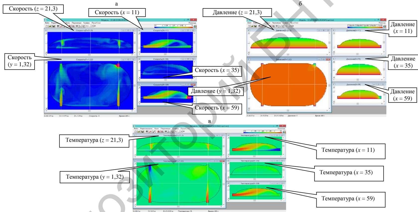
Рис. 5. Распределение расчетных параметров в момент времени 400 с в характерных сечениях при скорости поступления воздуха 5 м/с в полях: а – скоростей; б – давлений; в – температур
