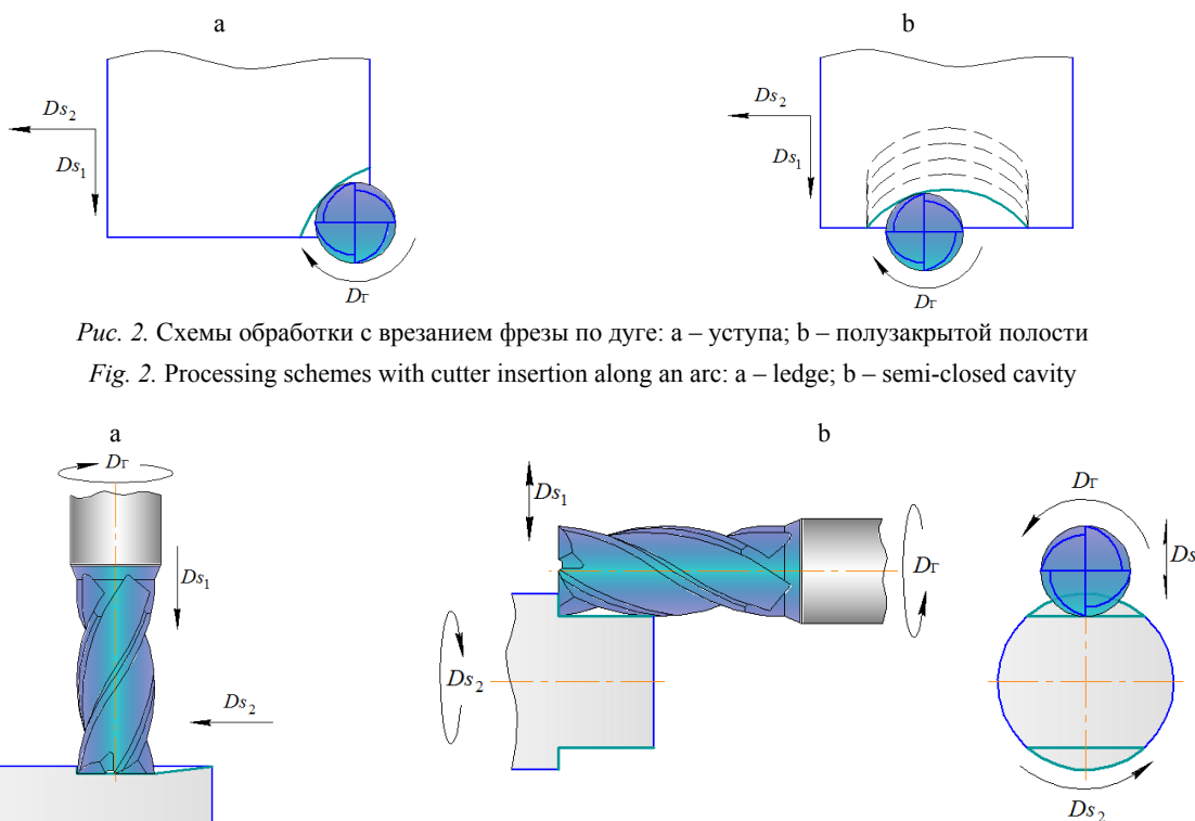
Рис. 3. Схемы обработки с врезанием фрезы по касательной: а – плоской поверхности детали; б – плоской и цилиндрической поверхностях детали
