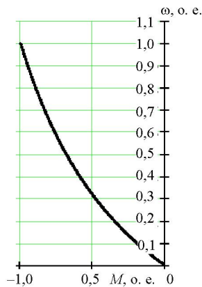
Рис. 3. Механическая характеристика муфты скольжения для двигателя АИР90
