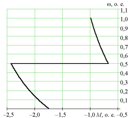
Рис. 4. Механическая характеристика АД с ВКТУ
