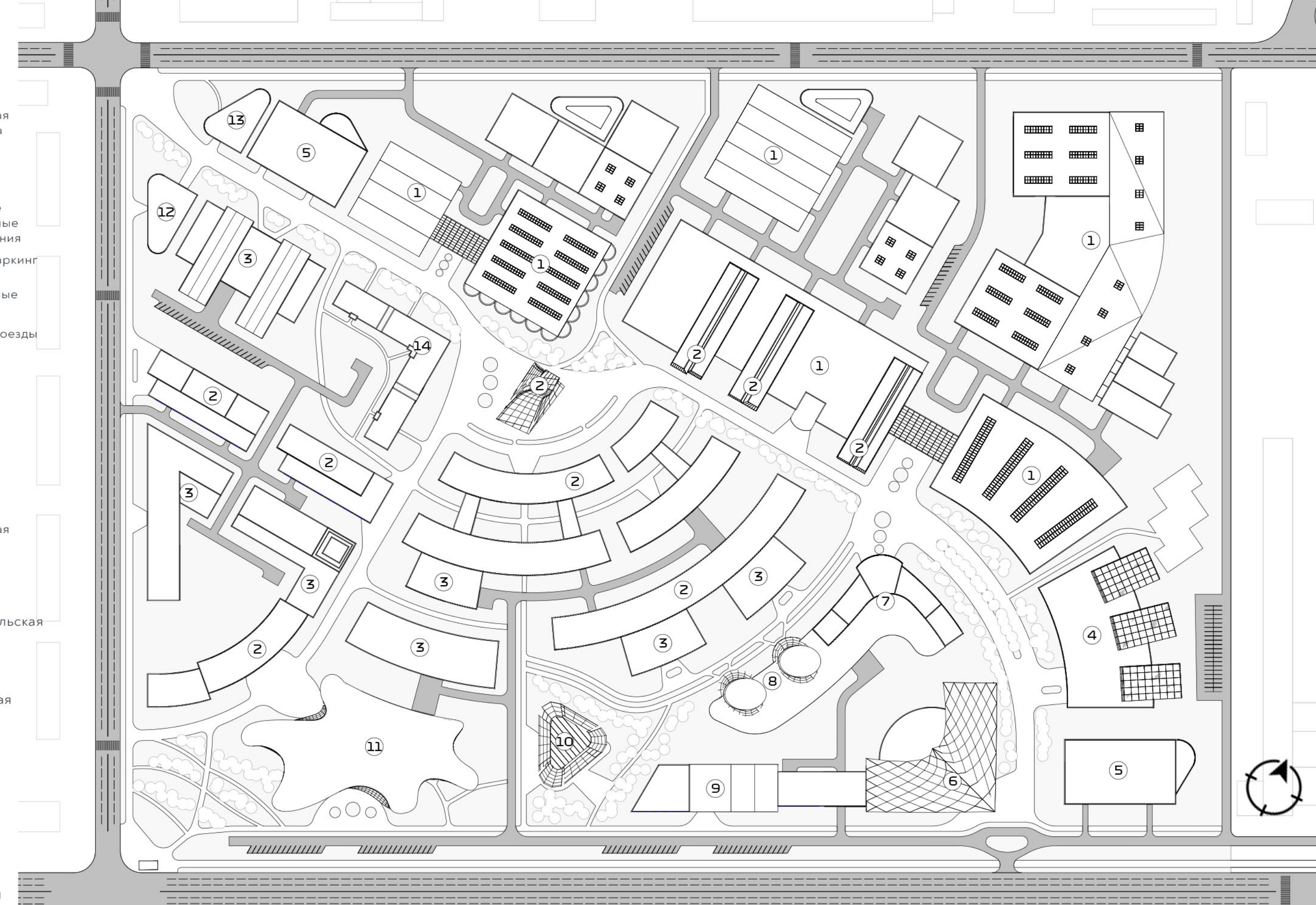
ГЕНПЛАН М 1:2000
