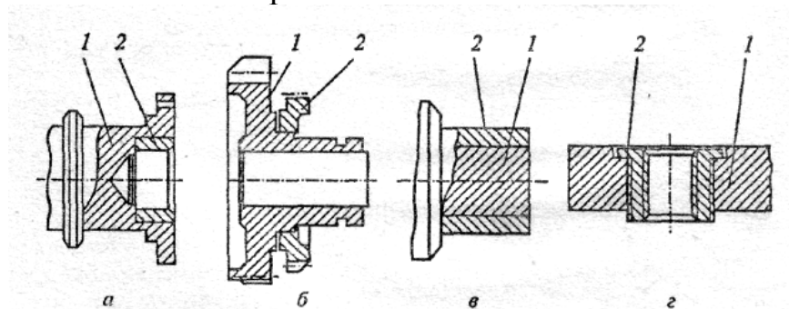
Рис. 4.3. Восстановление изношенных отверстий (а), шестерен (б), шеек цапф (в), резьбы (г) постановкой дополнительных деталей: 1 – изношенная деталь; 2 – дополнительная деталь
