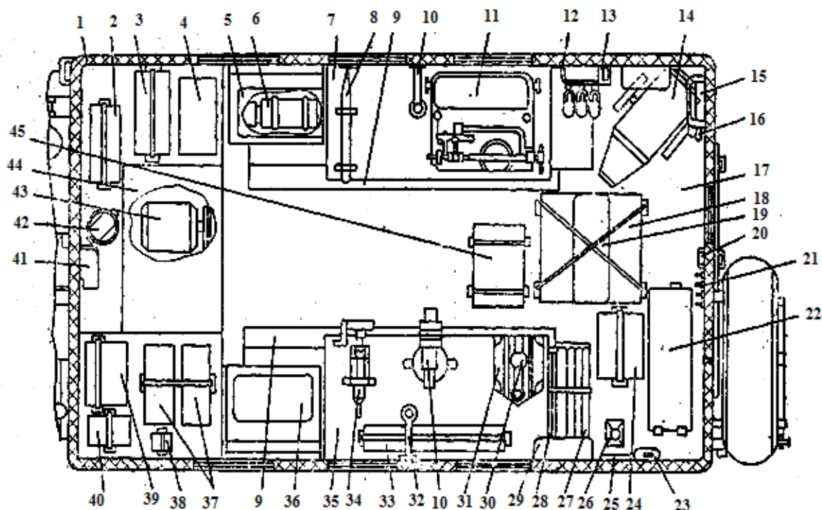
Рис. 2.5. Размещение оборудования и имущества в кузове мастерской MPC-AT-M1:
