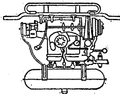
Рис. 2.29. Мотонасосный агрегат (мотопомпа), мод. МП-800Б
