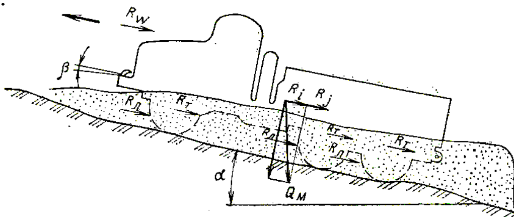
Рис. 3.1. Схема сил сопротивления движению объекта эвакуации:
