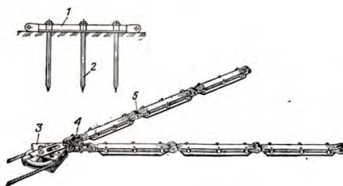
Рис. 3.25. Установка анкеров:
