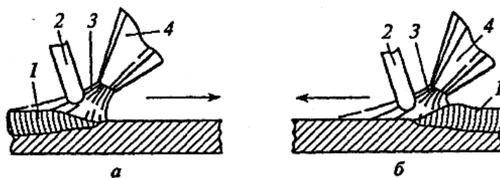
Рис. 4.11. Основные способы газовой сварки: а) правый; б) левый; 1 – формирующий шов; 2 – присадочный пруток; 3 – пламя горелки; 4 – горелка
