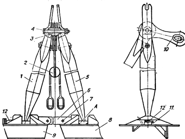
Рис. 3.24. Стрела-двунога:
