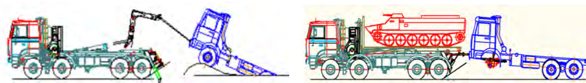
Рис. П13.2. Эвакуационная машина на базе МЗКТ-73011, оборудованная МПР-3 и устройством для транспортирования поврежденной техники полуподъемом
