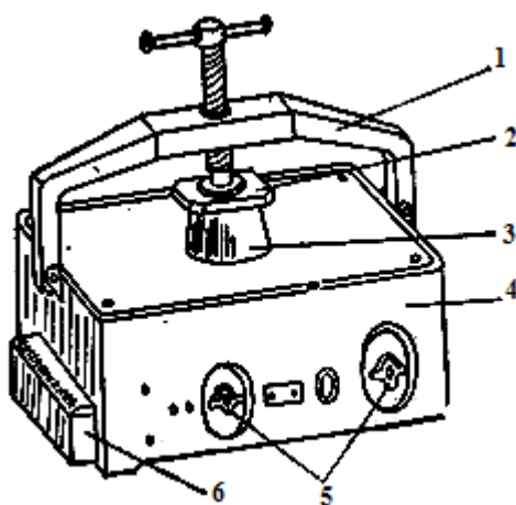
Рис. 2.28. Электровулканизационный аппарат:
