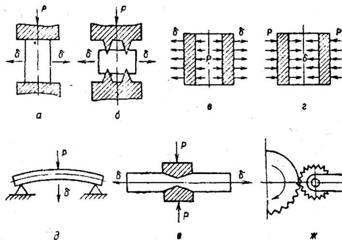
Рис. 4.8. Схема восстановления деталей пластическим деформированием: а – осадка; б – вдавливание; в – раздача; г – обжатие; д – правка; е – вытягивание; ж – накатывание; P – усилие деформации; δ – деформация
