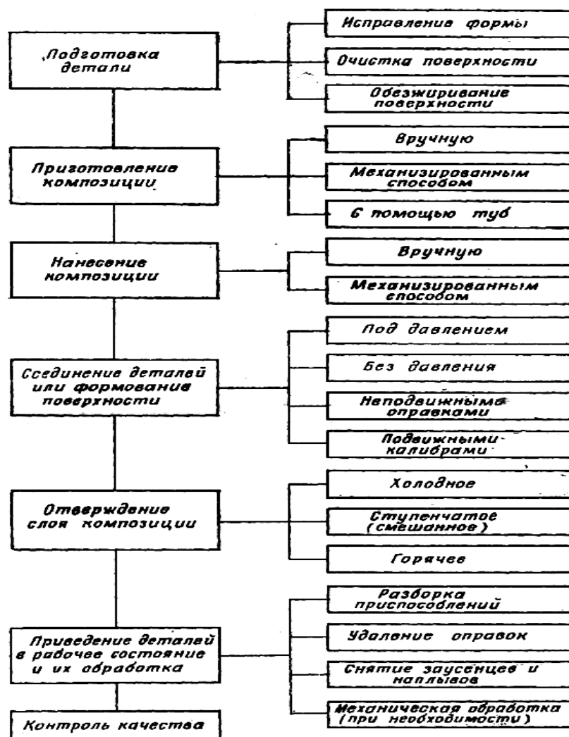
Рис. 4.12. Схема технологического процесса восстановления деталей эпоксидными композициями
