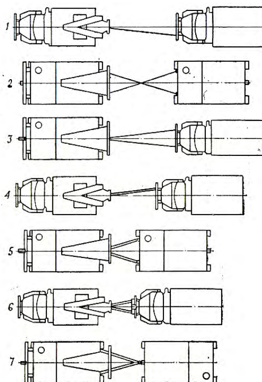
Рис. 3.40. Схемы и способы установки буксиров:
