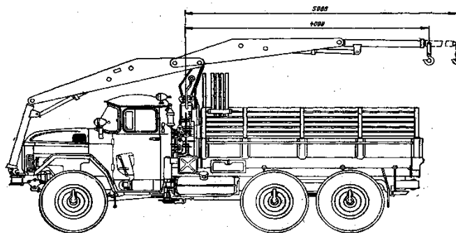
Рис. 2.39. Крановый самогрузчик 4901
