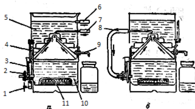
Рис. 2.20. Схема устройства дистиллятора: а – при наличии проточной водопроводной воды; б – при отсутствии проточной водопроводной воды; 1 – резиновый шланг; 2 – сливной кран; 3 – контрольная трубка; 4 – перепускная трубка; 5 – охладитель; 6 – резиновый сливной шланг; 7 – шланг для подачи воды от водопровода; 8 – резиновый перепускной шланг; 9 – отводная трубка; 10 – парообразователь; 11 – нагревательный элемент
