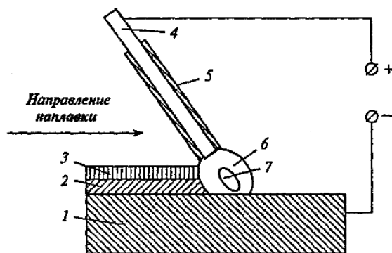
Рис. 4.10. Схема ручной электродуговой наплавки: 1 – основной металл; 2 – наплавленный валик; 3 – шлаковая корка; 4 – электродный стержень; 5 – покрытие электродного стержня; 6 – газшлаковая защита; 7 – сварочная ванна
