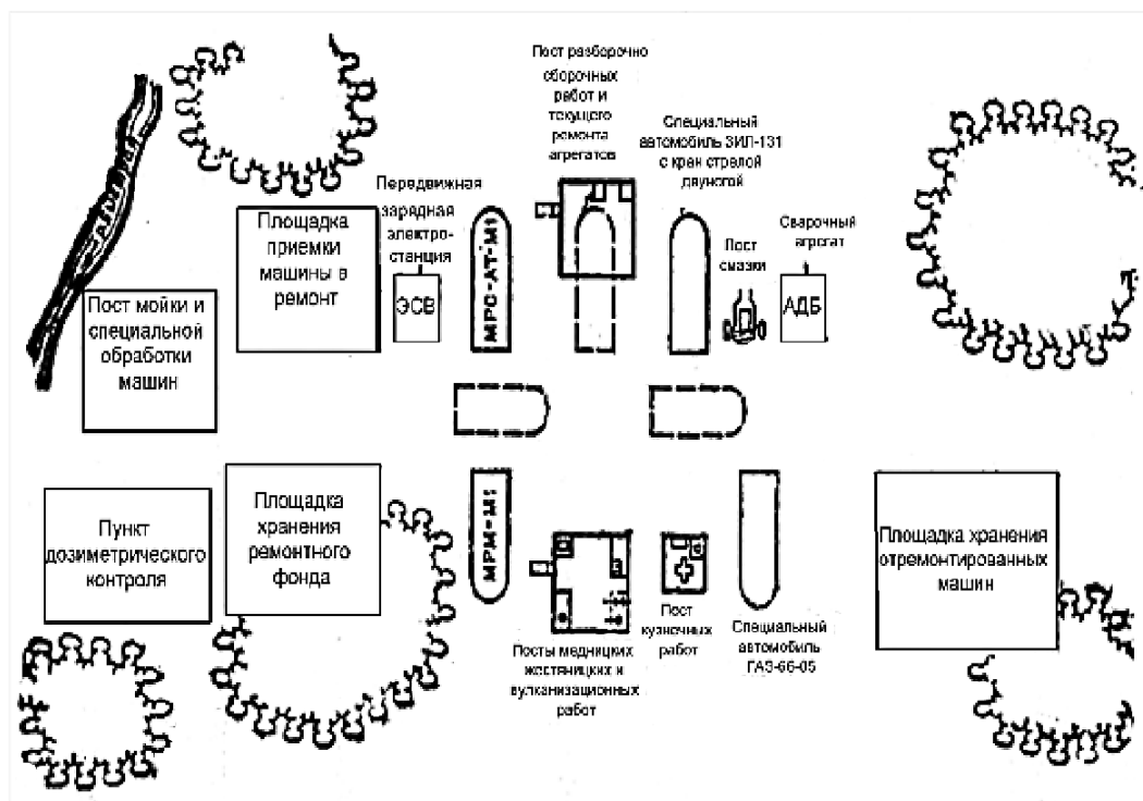
Рис. 2.47. Схема размещения на местности материальной части ПАРМ-1М1-4ОС (вариант 1)
