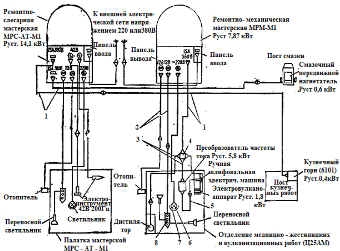
Рис. 2.21. Схема расположения кабельной электрической сети ПАРМ-1М1: 1 – кабель 25 мм (ВАРЭМ66-2506); 2 – кабель-удлинитель 12 В (Ц25А-2503); 3 – кабель ввода № 3 (ПМ1-2703); 4 – распределительная коробка 15-15 А (2502 А); 5 – кабель-удлинитель 36 В (ВАРЭМ66-2505 А); 6 – светильник с кабелем (Ц25 А-2502); 7 – свето-маскировочный колпак (П38-27); 8 – распределительная панель 12 В (ПМ5Л-2501 А)
