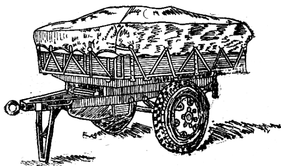
Рис. 2.17. Передвижная зарядная электростанция, мод. ЭСБ-4-ВЗ-1-М1, в походном положении
