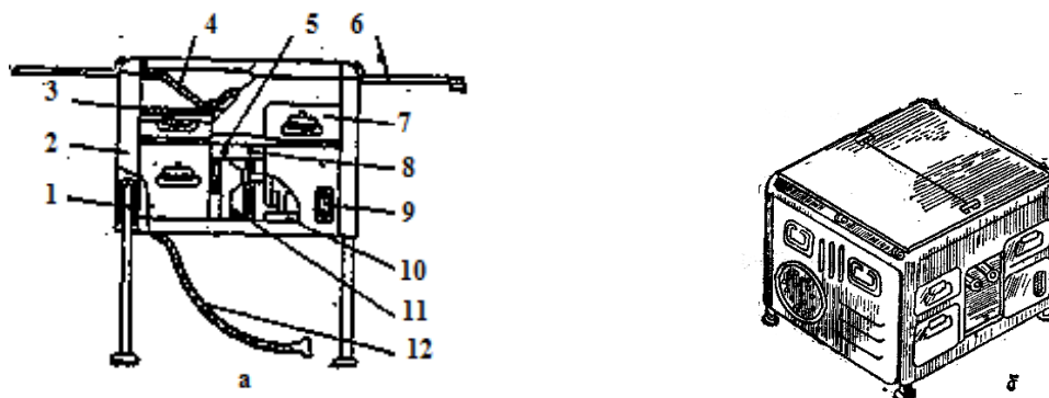
Рис. 2.33. Кузнечный горн: а – в рабочем положении; б – в транспортном положении;
