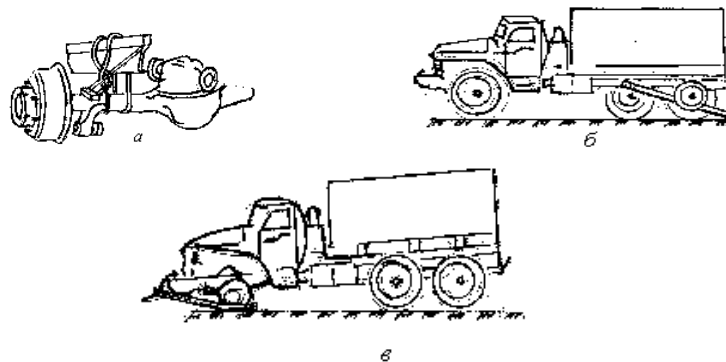
Рис. 3.39. Закрепление или снятие сорванных с мест крепления агрегатов и деталей, мешающих транспортированию объекта: а – подвязывание моста к лонжерону рамы; б – использование бревна для вывешивания моста; в – использование волокуши
