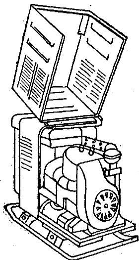
Рис. 2.18. Унифицированный бензоэлектрический агрегат
