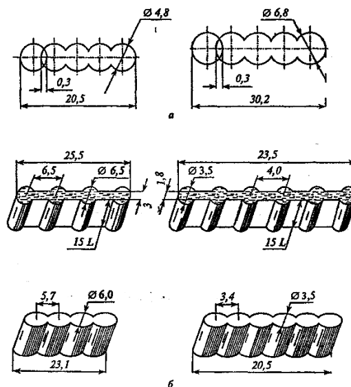
Рис. 4.4. Фигурные вставки: а – уплотняющие; б – стягивающие
