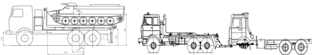
Рис. П13.1. Эвакуационная машина на базе МАЗ-6317, оборудованная МПР-3 и устройством для транспортирования поврежденной техники полуподъемом
