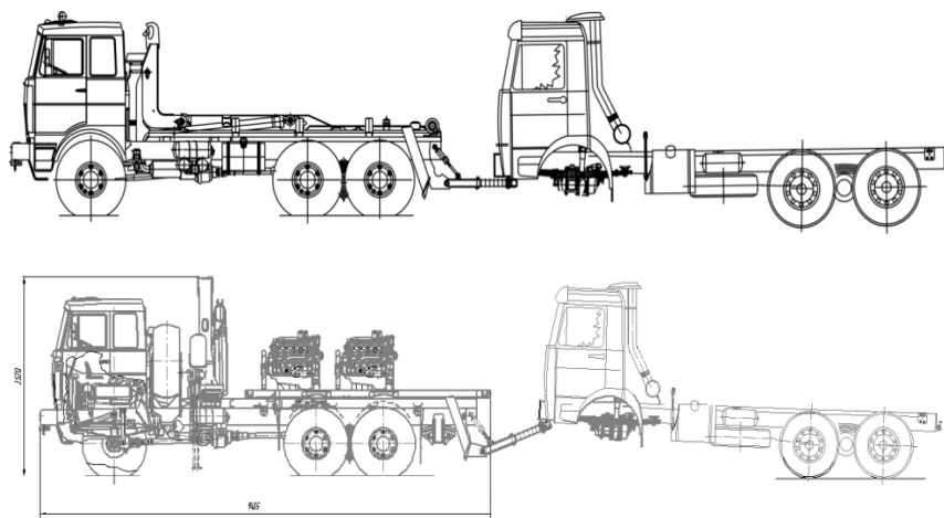
Рис. П7.5. Транспортировка поврежденной техники полуподъемом
