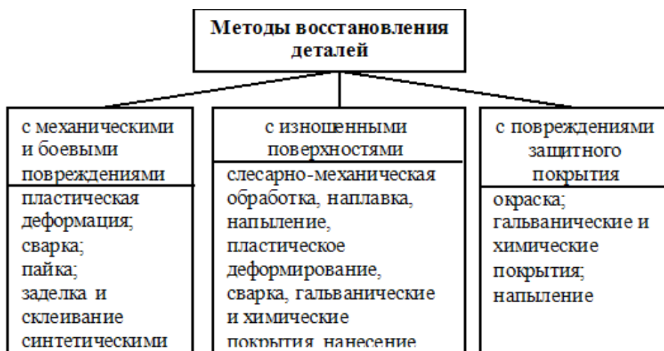
Рис. 4.2. Методы восстановления деталей
