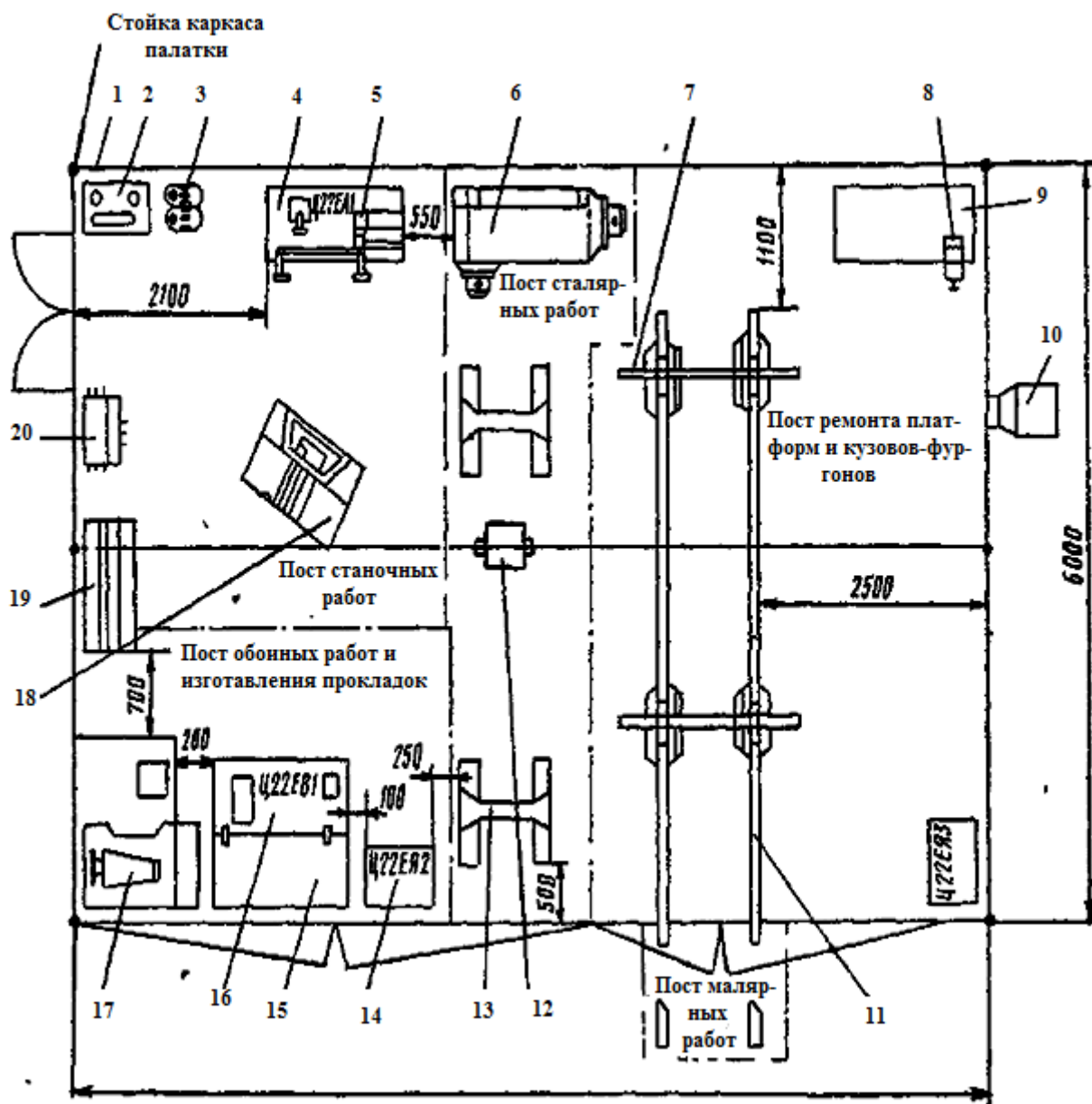
Рис. 2.44. Размещение оборудования отделения деревообделочных, обоечных и малярных работ Ц22Е:
