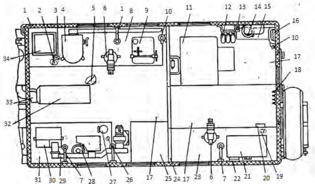
Рис. 2.35. Размещение оборудования и имущества в кузове мастерской проверки и ремонта автомобильного электрооборудования и приборов питания МЭСП-АТ-М1:
