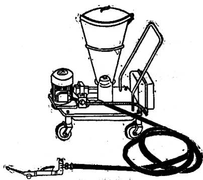
Рис. 2.30. Передвижной смазочный нагнетатель с электрическим приводом и бункером, мод. 390
