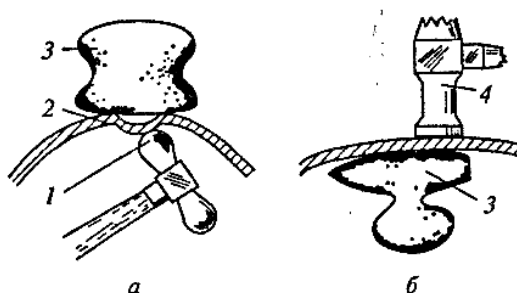
Рис. 4.9. Выколотка и рихтовка вмятин: а – выколотка; б – рихтовка; 1 – выколотка; 2 – вмятина; 3 – поддержка; 4 – рихтовальный молоток
