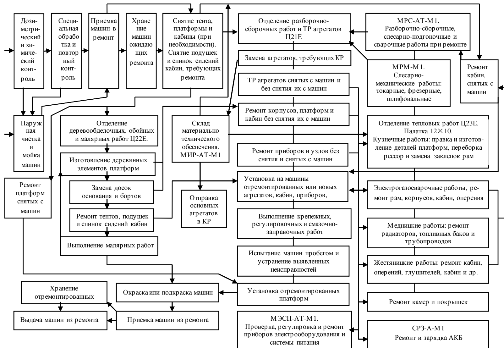
Рис. 5.3. Схема технологического процесса среднего ремонта машин в ПАРМ-3М1
