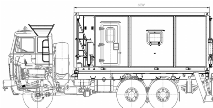
Рис. П7.1. Размещение кузова-контейнера с гидроопорами и устройства для транспортирования техники способом полупогрузки на шасси МАЗ-631705
