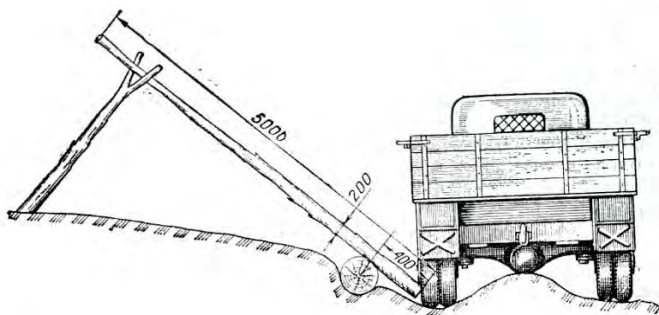
Рис. 3.17. Применение рычага при вытаскивании застрявшего автомобиля Величина фактического сопротивления перемещению при вытаскивании или транспортировании объектов зависит от способов их эвакуации.
