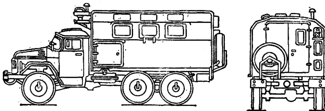
Рис. 2.4. Унифицированный кузов-фургон типа КМ131 или К131
