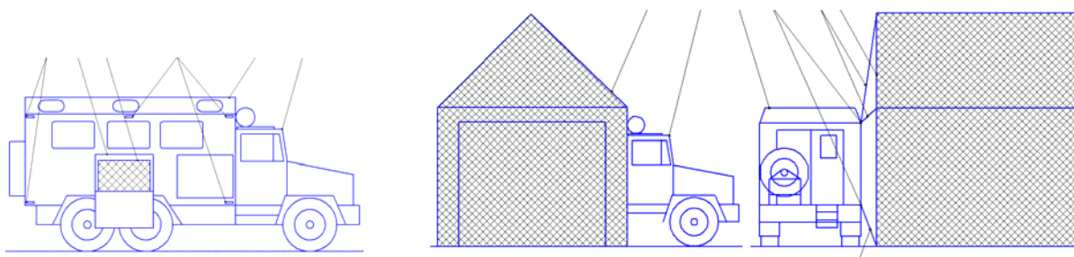
Рис. П7.7. Передвижная ремонтная мастерская с боковой каркасной палаткой
