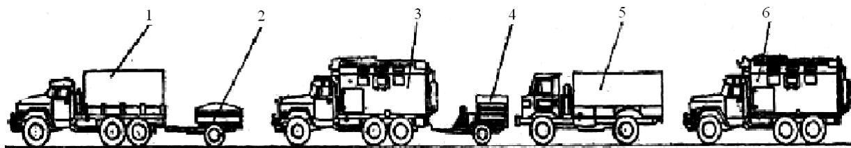
Рис. 2.50. Вариант построения колонны при перемещении ПАРМ-1М1-4ОС: 1 – специальный автомобиль ЗИЛ-131; 2 – передвижная зарядная электростанция; 3 – ремонтно-механическая мастерская МРМ-М1; 4 – сварочный агрегат на одноосном прицепе; 5 – специальный автомобиль ГАЗ-66-05; 6 – ремонтно-слесарная мастерская МРС-АТ-М1
