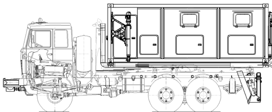
Рис. П7.2. Съемный кузов-контейнер постоянного объема
