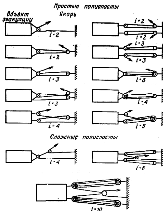
Рис. П9.1. Схема простых и сложных полиспастов из одно – и двух роликовых блоков
