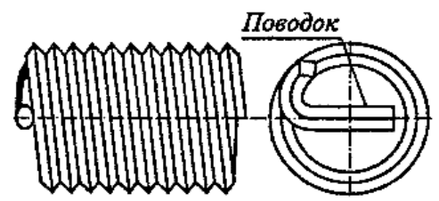
Рис. 4.6. Резьбовая спиральная вставка
