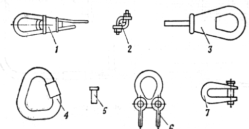
Рис. 3.26. Соединительные детали такелажного оборудования
