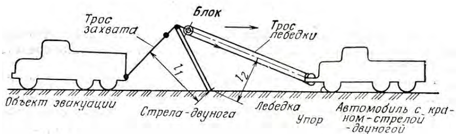
Рис. 3.16. Схема применения стрелы-двуноги при вытаскивании объекта
