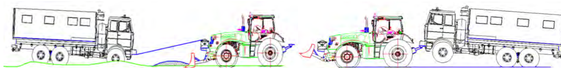
Рис. П13.4. Эвакуационная машина на базе колесного трактора «Беларус 3023» с электромеханической трансмиссией, дооборудованного земляным отвалом, гидравлической лебедкой и устройством для транспортирования поврежденной техники полуподъемом
