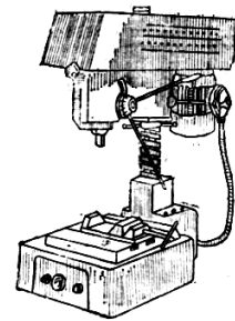
Рис. 2.14. Настольно-сверлильный станок, мод. 2М112-BC327
