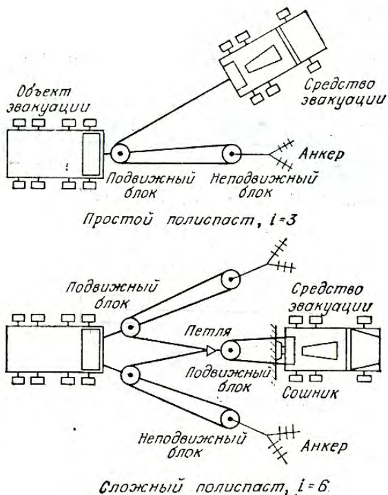
Рис. 3.15. Принципиальные схемы простого и сложного полиспаста
