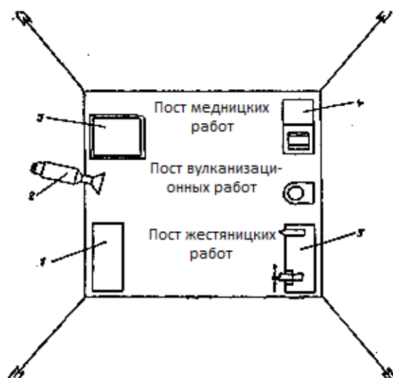
Рис. 2.23. Размещение оборудования постов отделения медницко-жестяницких и вулканизационных работ в палатке: 1 – слесарный верстак; 2 – отопительная установка; 3 – ванна для проверки радиаторов и камер; 4 – выносной стол с электровулканизационным аппаратом; 5 – слесарный верстак с тисками и оправкой для жестяницких работ
