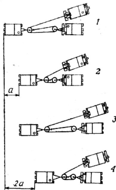
Рис. 3.38. Применение подвижного анкера для растягивания полиспастов:
