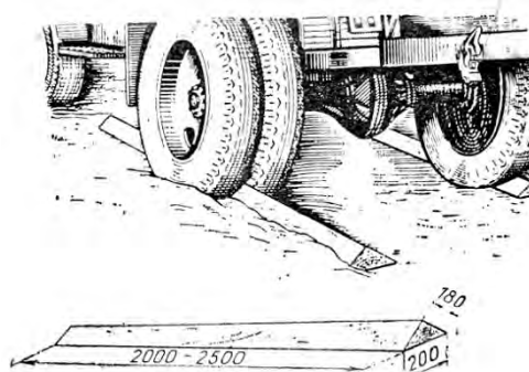
Рис. 3.29. Применение брусьев для самовытаскивания
