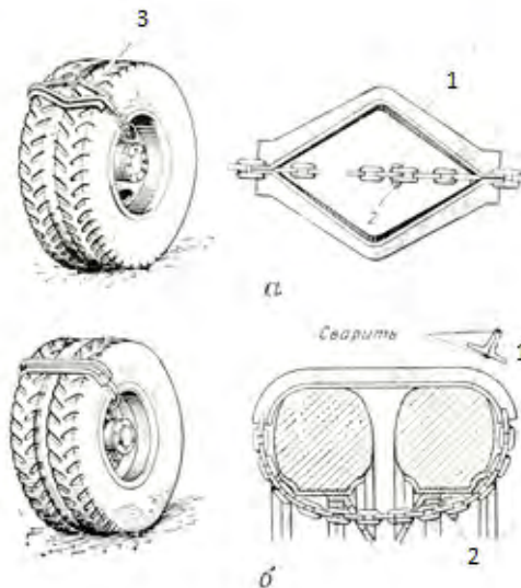
Рис. 3.9. Противобуксовочная колодка: а – ромбовидная; б – прямая; 1 – уголок (50×50×5); 2 – замок; 3 – колодка в сборе
