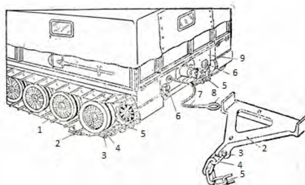
Рис. 3.11. Установка башмаков под гусеницы для работы лебедки транспортера-тягача: 1 – гусеница; 2 – башмак; 3 – валик; 4 – серьга; 5 – цепь; 6 – буксирный крюк; 7 – трос лебедки; 8 – коуш; 9 – корма
