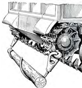
Рис. 3.32. Крепление бревна буксирным тросом при самовытаскивании
