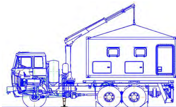
Рис. П7.4. Снятие кузова-контейнера мастерской МРС-АТБ
