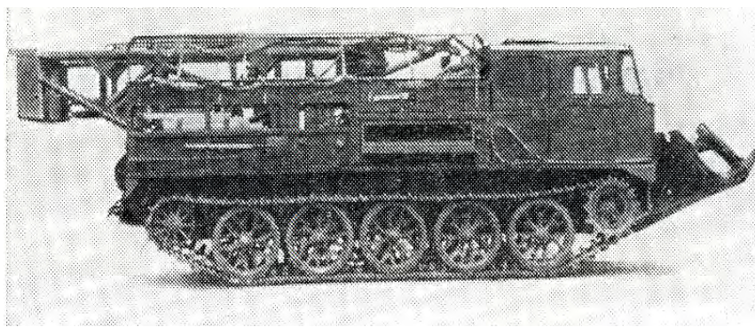
Рис. 3.21. Средний гусеничный эвакуационный тягач ГЭТ-С модели ТГ4
