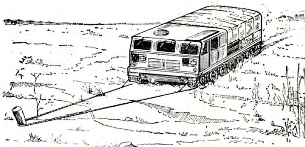
Рис. 3.33. Самовытаскивание с использованием тросов, закрепленных за гусеницы
