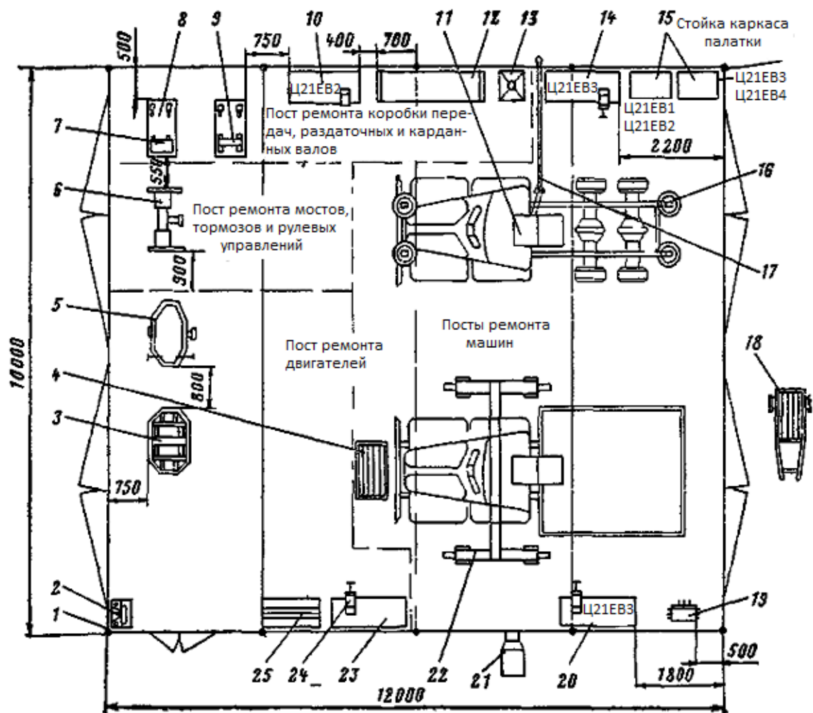
Рис. 2.41. Размещение оборудования отделения разборочно-сборочных работ и текущего ремонта агрегатов Ц21Е:
