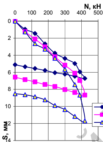
Рисунок 4. – Графики зависимости «осадка-нагрузка» для свай Ø 325 мм
