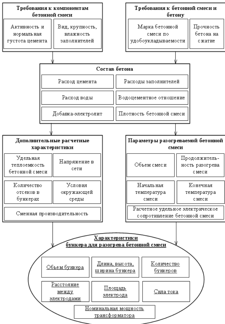
Рис. 1. Последовательность расчета параметров электроразогрева бетонной смеси
