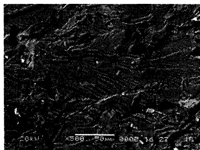
Рис. 4. Усталостный излом сплава, полученного с использованием рафинирующе-модифицирующего комплекса при частоте испытаний 0,3 кГц. ×500
