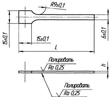
Рис. 1. Геометрические параметры образца для усталостных испытаний
