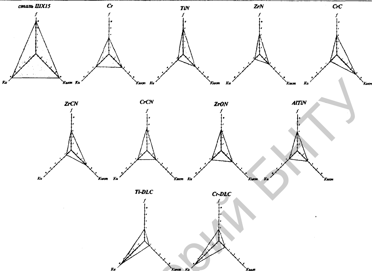
Рис. 1. Симплекс триботехнических свойств покрытия
