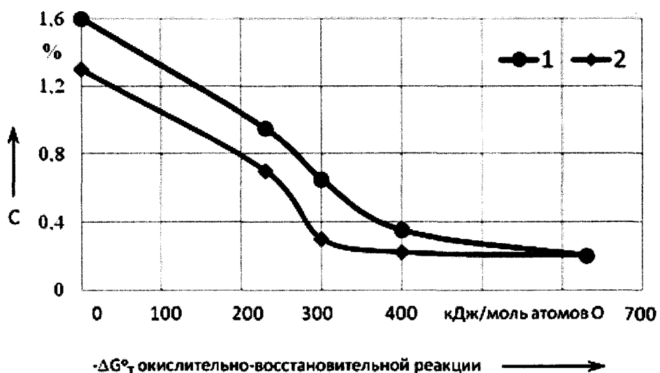
Рис. 2. Влияние величины -\Delta G^{\circ}_T окислительно-восстановительной реакции, протекающей в композициях «Cu–Al (2,4 %)–легирующий оксид», на концентрацию Al в твердом растворе после механического легирования (1); механического легирования и отжига (2)
