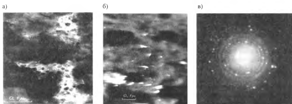
Рис. 3. Микроструктура гранул, полученных обработкой в течение 8 ч в механореакторе композиции «Cu–Al (0,80 %)– \text{MoO}_3 (2,13 %)). ПЭМ: а – светлое поле; б – темное поле в рефлексах фаз [111]\text{Cu} + [111]\text{Al} ; в – микроэлектронграмма
