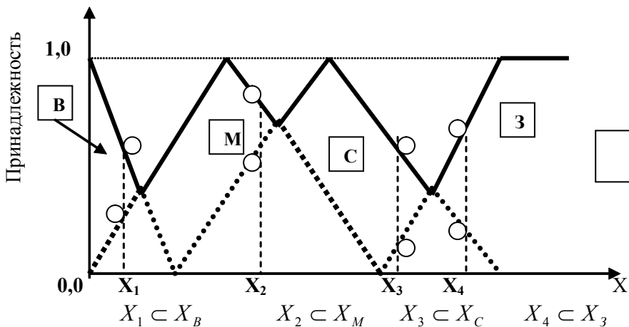
Рис.2 - Определение принадлежности значения X_i одной из лингвистических переменных О, М, С или З.
