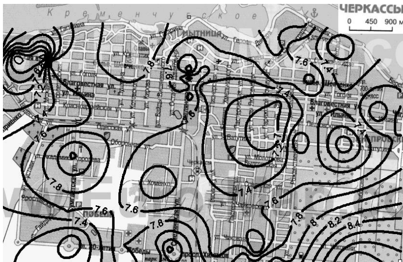
Рис. 1 – Карта кислотности ( pH_{\text{вод.}} ) почв г. Черкассы
