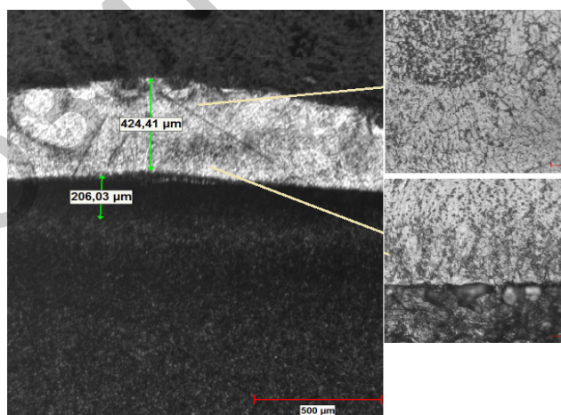
Рис. 2. Микроструктура контрольного образца стали марки 20X13
