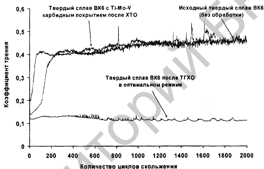
Рис. 5. Сравнительная диаграмма изменения коэффициента трения твердого сплава ВК6 до и после упрочнения. Условия испытаний: сухое трение, нагрузка 1 Н, длина хода (трека) 3 мм, скорость 4 мм/с; оптимальный режим ТГХО: ХО в составе TiO_2-MoO_3 при T = 100^\circ C , \tau = 19 мин; ТО при T = 1035^\circ C , \tau = 10 мин
