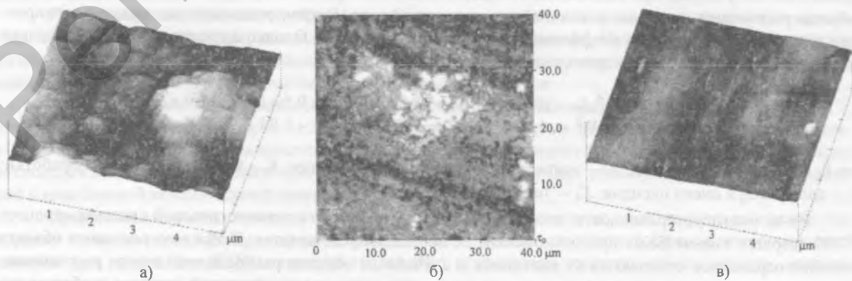
Рис. 3. Морфология поверхности твердого сплава ВК6, подвергнутого ТГХО, до (а, б) и после испытаний на трение (в) режим ТГХО:
