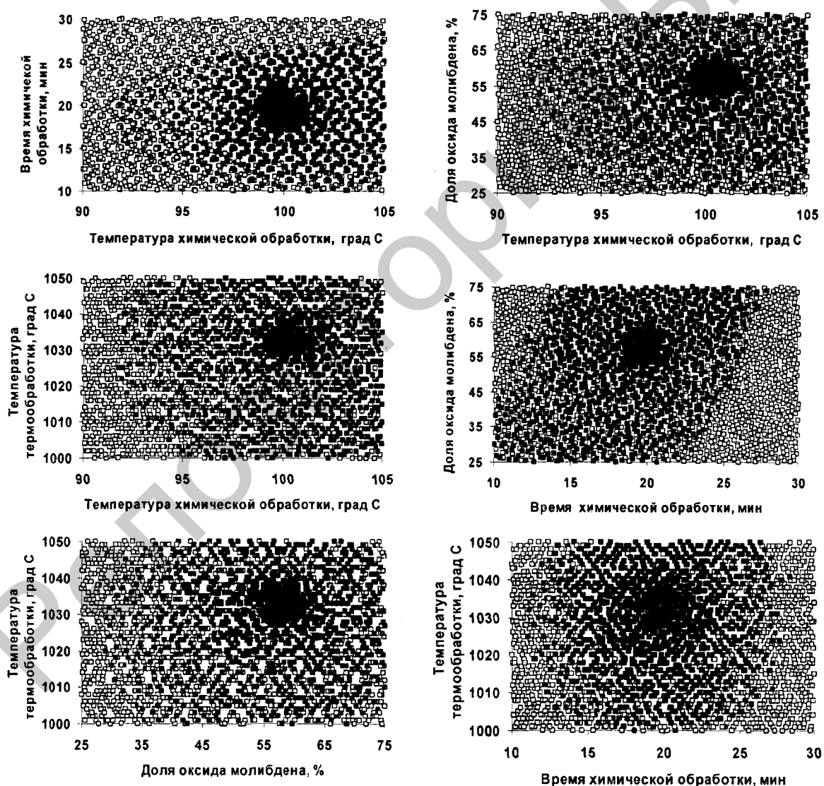
Рис. 4. Дискретные портреты виртуального пространства технологической системы процесса ТГХО твердого сплава ВК6 в вододисперсном составе на основе TiO 2 -MoO 3 :
