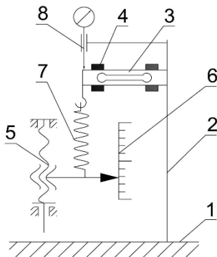
Рисунок 1. Схема принципиальная для исследования упругих характеристик пружин растяжения
