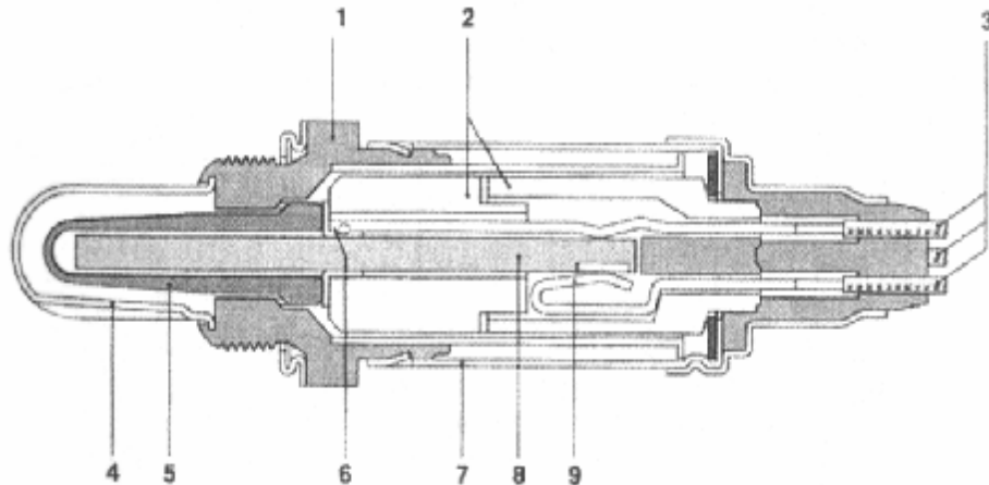
Рис. 3.19 Датчик концентрации кислорода ( \lambda –зонд)
