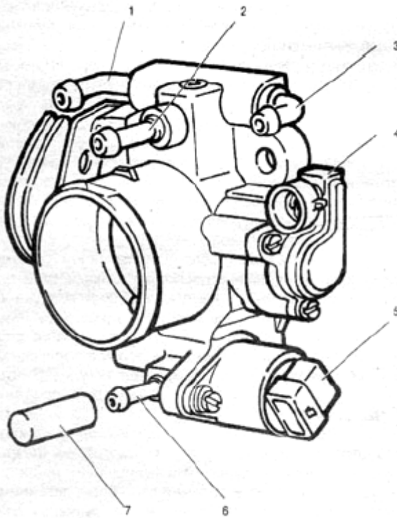
Рис.4.6. Дроссельный патрубок
