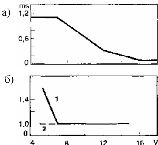
Рис. 3.37. Функции компенсации напряжения: 1-насос поточного типа; 2-насос с принудительным смещением
