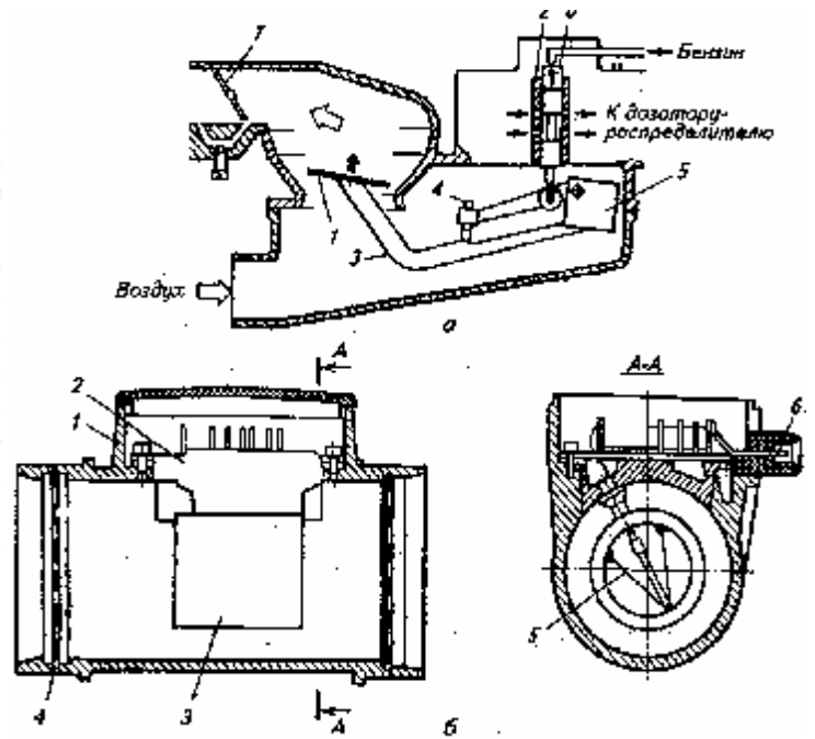
Рис. 4.9 Датчики расхода воздуха
