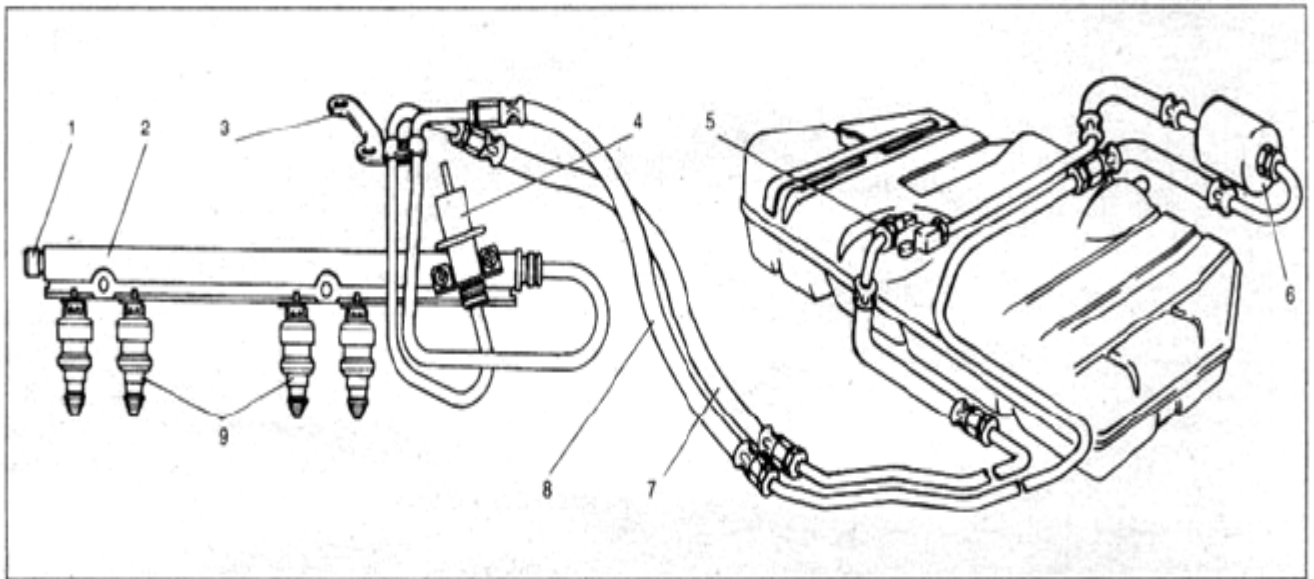
Рис. 4.4. Система подачи топлива:
