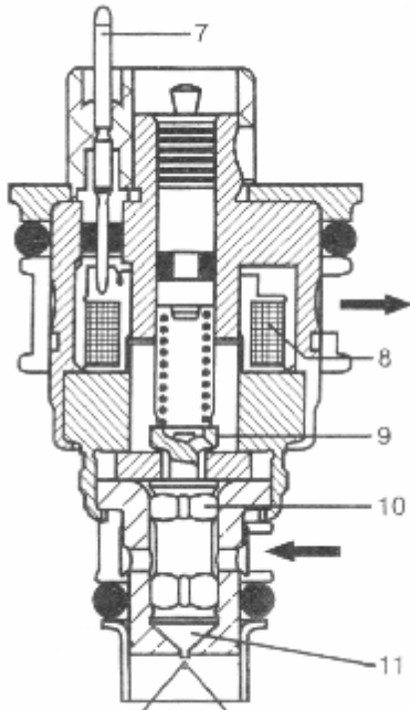
Рис. 3.8. Электромагнитная форсунка
