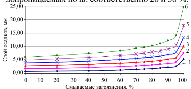
Рис. 1. Зависимость расчетного критического слоя осадков от процента смываемых загрязнений при различных значениях удельного веса площади водопроницаемых почв в общей площади водосбора для k_c = 0,0045 : 1 – 0; 2 – 20; 3 – 40; 4 – 60; 5 – 80; 6 – 100 %
