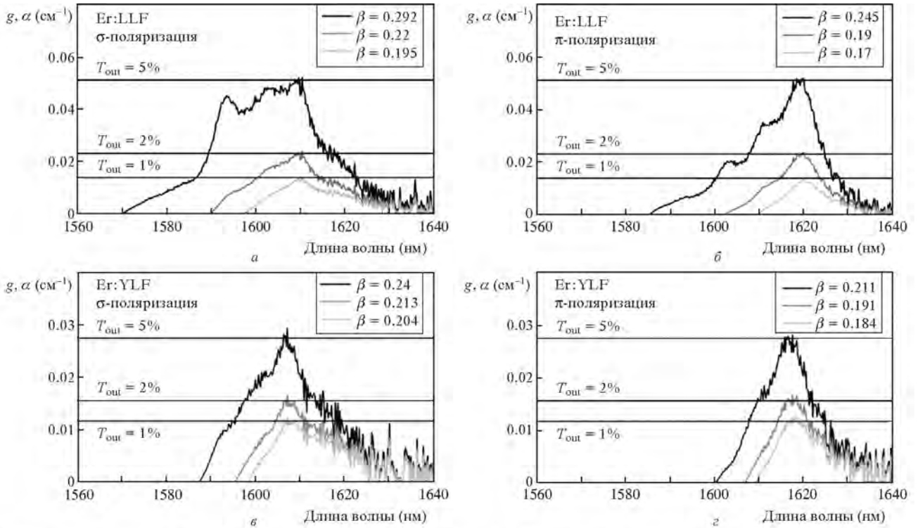
Рис.3. Спектры усиления g(\lambda) кристаллов Er:LLF (а, б) и Er:YLF (в, г) для \sigma - (а, в) и \pi - (б, г) поляризаций излучения с указанием уровня внутрирезонаторных потерь \alpha (прямые линии) при различных значениях пропускания выходного зеркала T_{out} .
