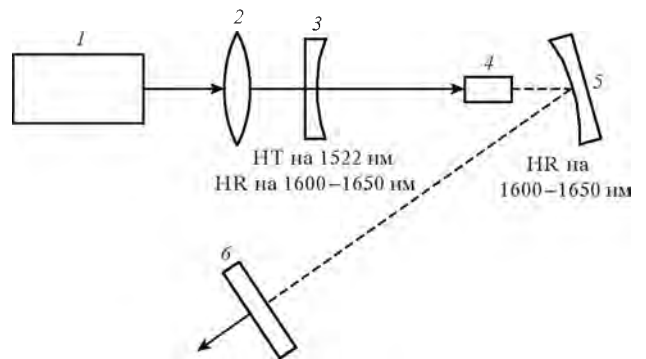
Рис.4. Схема лазера: 1 – твердотельный лазер ( \lambda_p = 1522 нм); 2 – система фокусировки; 3 – входное сферическое зеркало ( R = -150 мм); 4 – активный элемент (Er:LLF или Er:YLF); 5 – сферическое зеркало ( R = -75 мм); 6 – выходное зеркало ( T_{out} = 1\%, 2\%, 5\% ).
