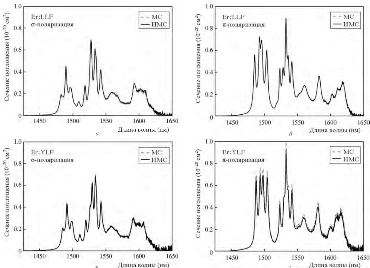
Рис.2. Спектры поперечных сечений стимулированного излучения кристаллов Er:LLF (а, б) и Er:YLF (в, г) для \sigma - (а, в) и \pi - (б, г) поляризации излучения.
