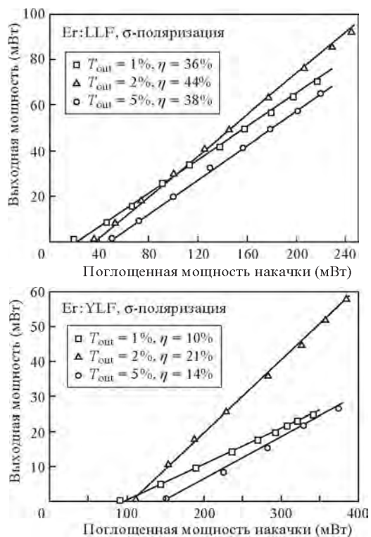
Рис.5. Выходные характеристики лазеров на кристаллах Er:LLF (а) и Er:YLF (б).
