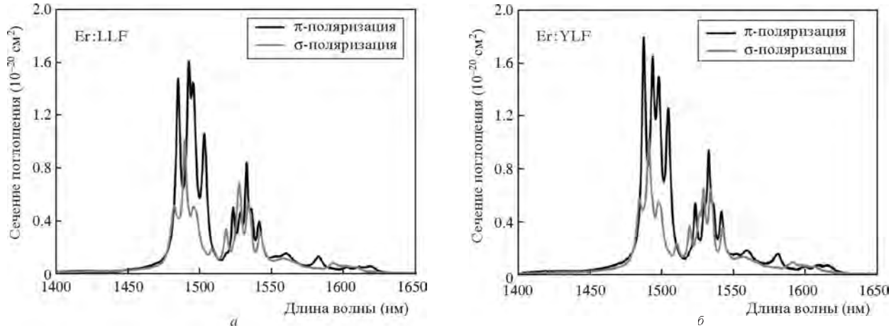
Рис.1. Спектры поперечных сечений поглощения кристаллов Er:LLF (а) и Er:YLF (б).
