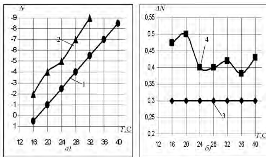
Рис. 4 Влияние конфигурации в плане (а) и толщины (б) пенополиуретановой полировальной подложки на общую N и местную \Delta N погрешность формы оптических поверхностей при доводке притирами с различной формой полировальных подложек: 1 – полировальная подложка толщиной 1 мм с искривленными каналами СОЖ; 2 – подложка толщиной 1 мм с прямыми каналами СОЖ; 3 - полировальная подложка толщиной 1 мм с искривленными каналами СОЖ; 4 - полировальная подложка толщиной 0,5 мм с искривленными каналами СОЖ
