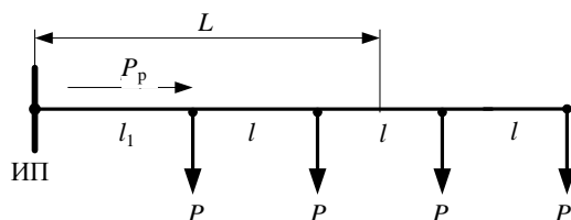
Рис. 1. Схема групповой линии электрического освещения с равномерно распределенной нагрузкой: ИП – источник питания (ОЩ) Fig. 1. The pattern of a group line of electric lighting with evenly distributed load: IP – power supply
