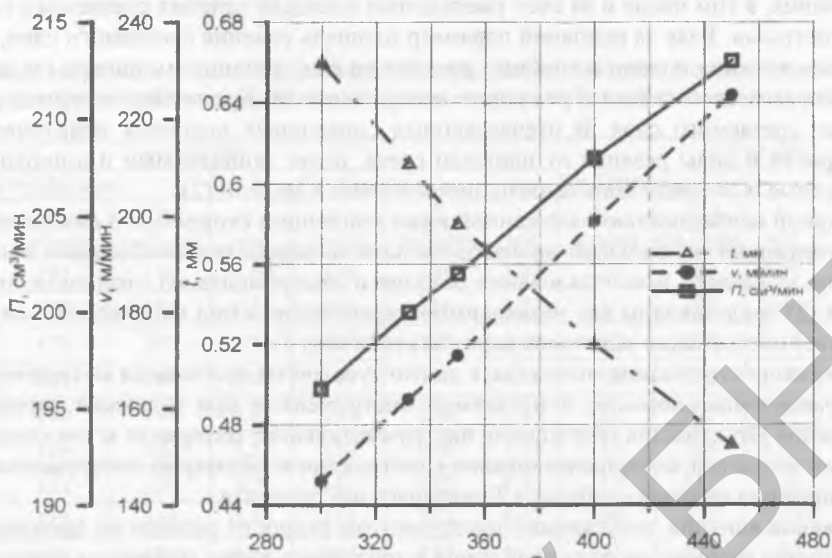
Рис. 1. Зависимость v , P и t от коэффициента C_v при полной загрузке станка по мощности ( N = 10 кВт) и фрезы по стойкости ( T = 90 мин) для твердого сплава T15K6 при S_z = 0,8 мм/зуб
