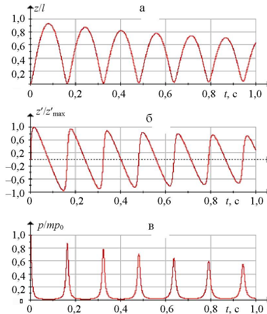
Рис. 2. Пульсации продуктов газового взрыва в открытой снизу недеформируемой цилиндрической взрывной камере: а – z/l = f(t) ; б – z'/z'_{\max} = f(t) ; в – p/mp_0 = f(t) при R_1 = 0,10 м; R_\phi = 0,12 м; R_K = 0,12 м; L_\phi = 10 м; L_K = 60 м; a = 0 ; l = 1 м; h = 0,1 м; h_1 = 0,05 м; m = 10 ; n = 1,9 . Вычисленные значения: Z'_{\max} = 3,87 м/с при Z_M = 22,7 см; Z_{\max} = 93,3 см
