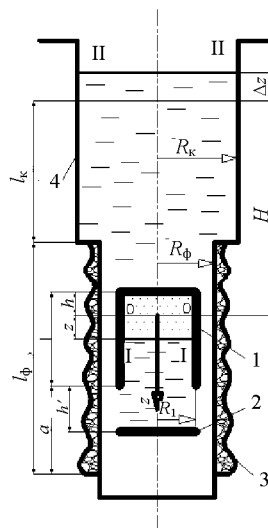
Рис. 1. Расчетная схема пульсаций продуктов газового взрыва в открытой снизу недеформируемой цилиндрической взрывной камере, находящейся в скважине: 1 – взрывная камера; 2 – отражатель; 3 – фильтр; 4 – колонна
