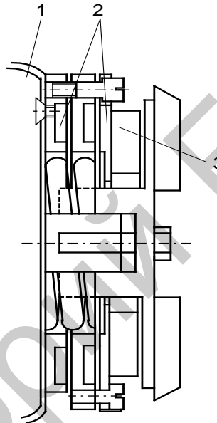
Рис. 3. Встраиваемый электромеханический тормоз с увеличенным ходом якоря:
