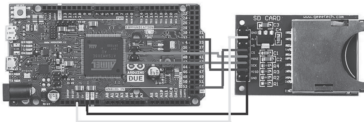
Рис. 1. Общий вид ArduinoDue с SD модулем и схема их соединения
