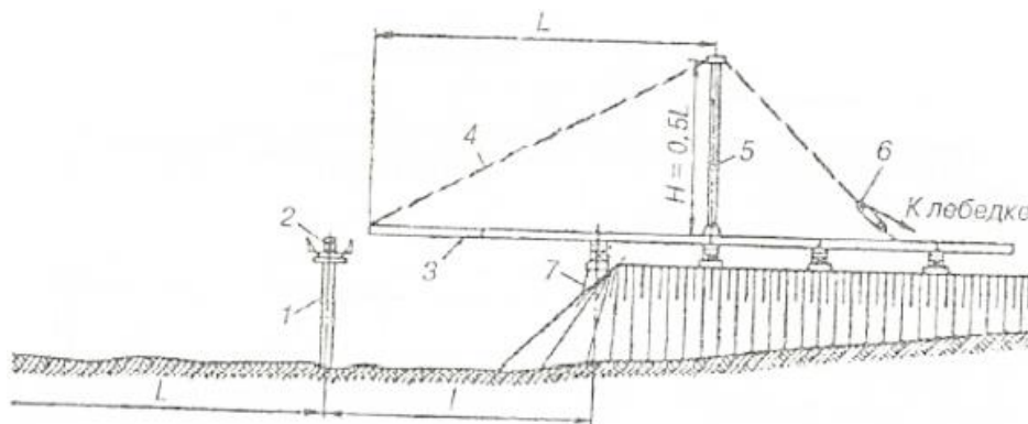
Рис. 2. Шпренгель:
