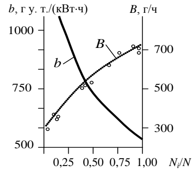
Рис. 5. Удельный ( b ) и массовый ( B ) расходы топлива теплоэнергетической установкой
