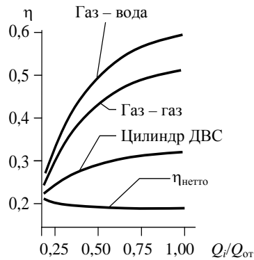
Рис. 4. Изменение эффективности (коэффициента использования теплоты топлива) микроТЭС в зависимости от отопительной нагрузки
